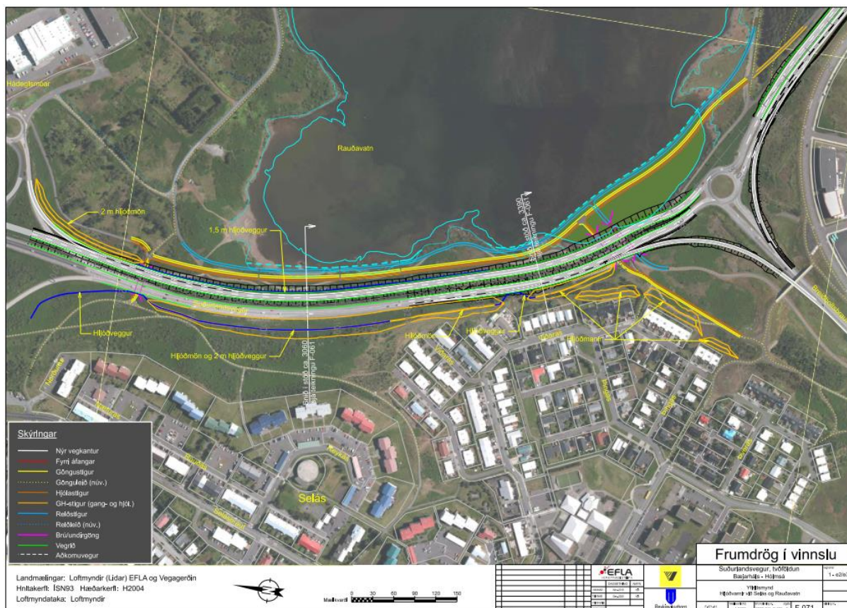
MYND 5.51 Yfirlitsmynd af hljóðvörnum við Selás og Rauðavatn (teikning EFLA, 2021).
