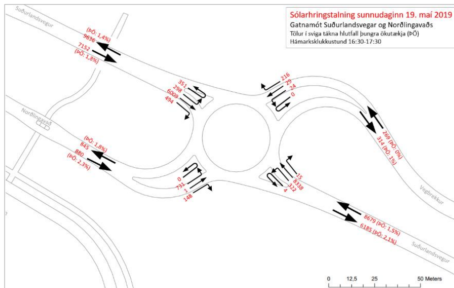
MYND 3.17 Sólarhringsumferð við Norðlingavað sunnudaginn 19. maí 2019 skv. talningum EFLU.
