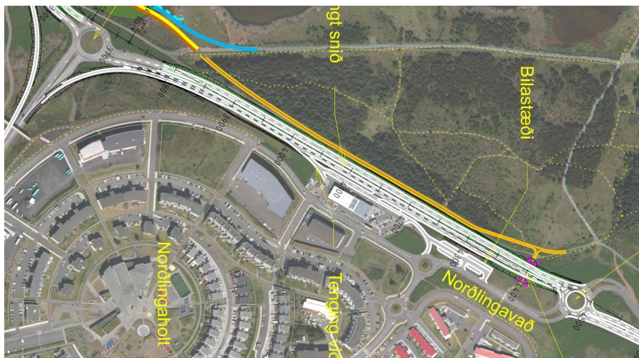
MYND 5.53 Breikkun 1. áfanga Suðurlandsvegur frá Breiðholtsbraut að Norðlingavaði í mjóu sniði.
