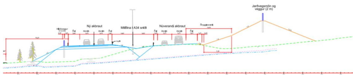
MYND 5.43 Hljóðvarnir í sniði 1, stöð 3060. Grænt er núverandi landhæð, gult er ný hljóðvörn. Fleiri snið eru í teikningahefti.
