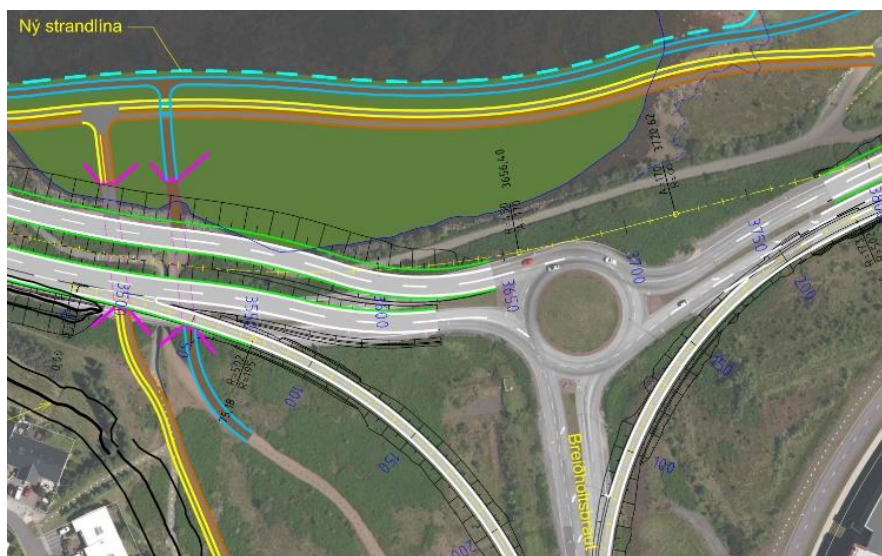
MYND 3.14 Tvöföldun Suðurlandsvegur tengd í núverandi hringtorg við Breiðholtsbraut í áfanga 1.
