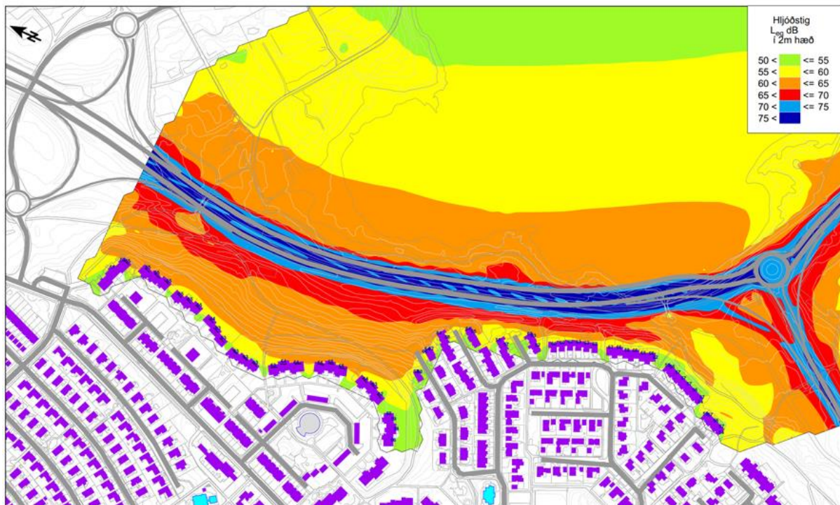
MYND 5.42 Hljóðstig frá umferð á tvöföldum vegi við Seláshverfi (stærri mynd í viðauka I).
