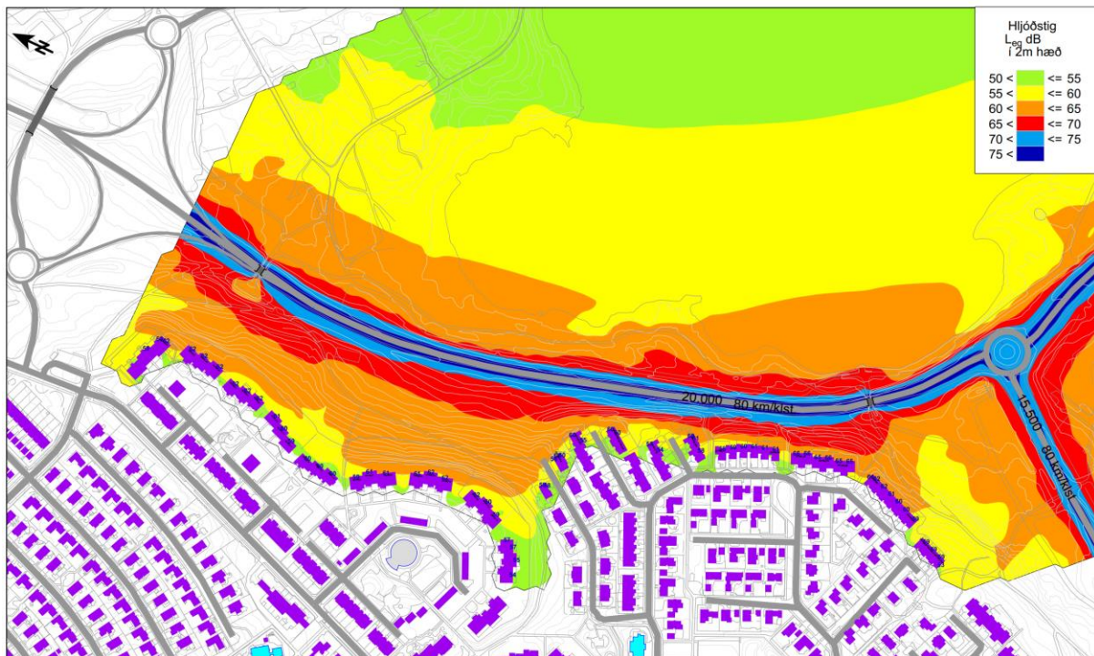
MYND 5.41 Hljóðstig frá umferð á núverandi vegi við Seláshverfi (stærri mynd í viðauka I).
