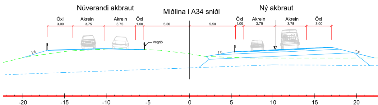
MYND 3.11 Þversnið Suðurlandsvegar, almennt.
