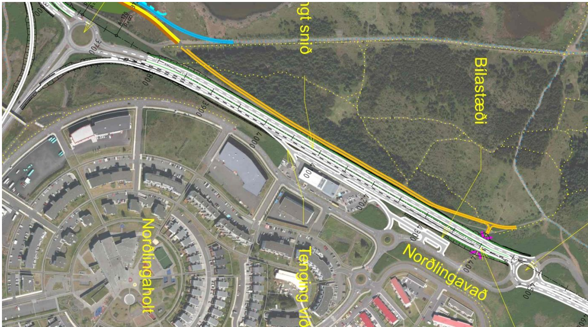
MYND 3.9 Breikkun 1. áfanga Suðurlandsvegar frá Breiðhóltsbraut að Norðlingavaði í mjóu sniði.
