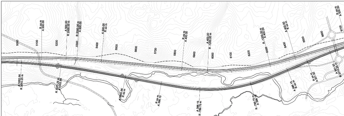
MYND 3.2 Nyrðri akbraut Suðurlandsvegur lögð fyrir norðan Hólmsá (frumdrög 2002).
