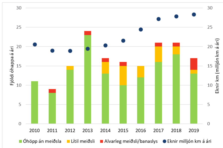
MYND 5.63 Umferðaróhöpp á Suðurlandsvegi 2010-2019, frá vegamótum við Bæjarháls að Hólmsá, ásamt fjöldi ekinna km
