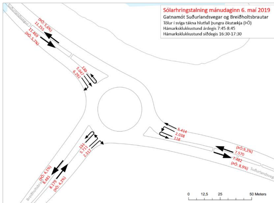
MYND 3.15 Sólarhringsumferð á vegamótum við Breiðholtsbraut mánudaginn 6. maí 2019 skv. talningum EFLU.
