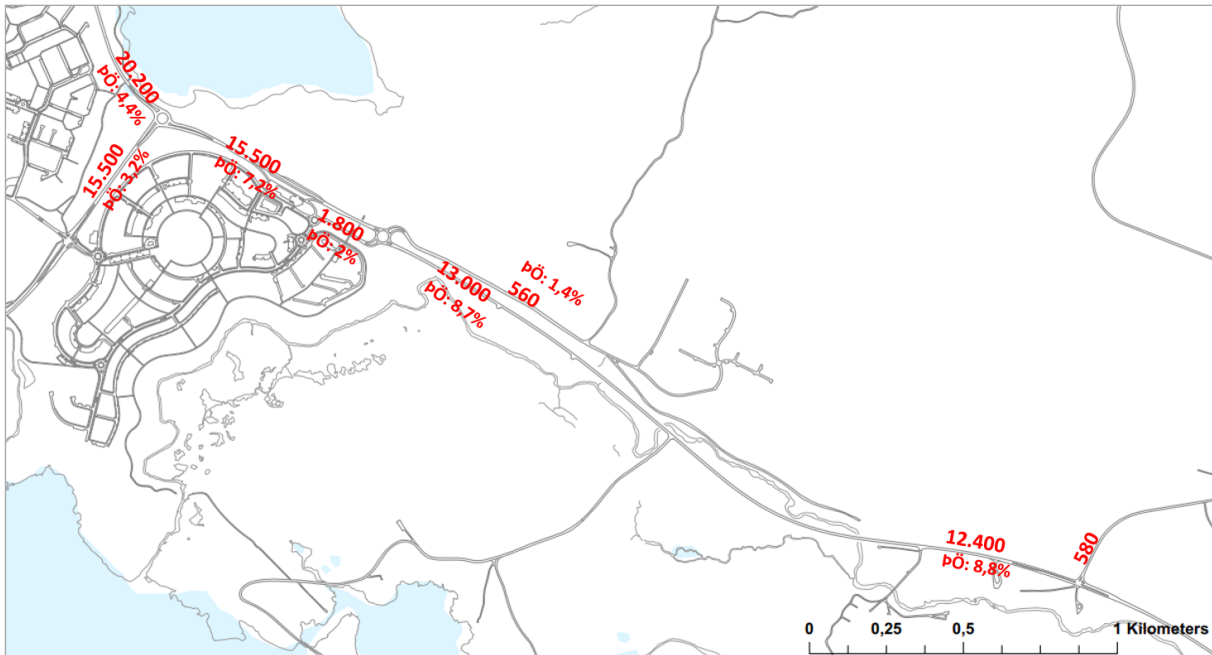
MYND 5.61 Áætluð ársdagsumferð (ÁDU) 2018 á Suðurlandsvegi, Breiðholtsbraut og nágrenni, ökutæki á sólarhring, auk hlutfalli þunga ökutækja (PÖ).
