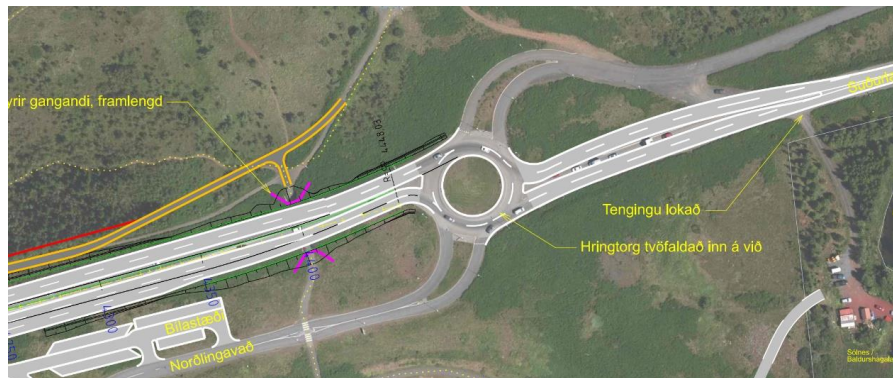
MYND 3.16 Breikkað hringtorg við Norðlingavað í áfanga 1.
