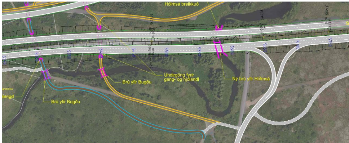
MYND 3.20 Lausn 2 af tengingu Heiðmerkurvegjar við Suðurlandsveg.
