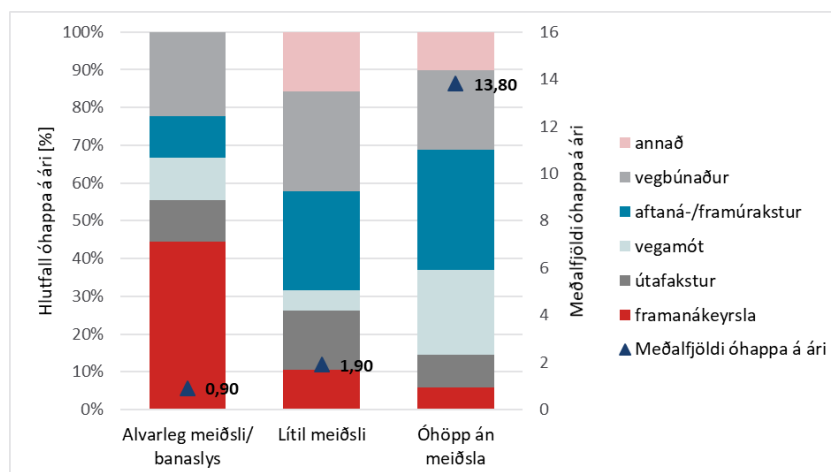
MYND 5.64 Meðalfjöldi umferðaróhappa á ári á Suðurlandsvegi frá Bæjarhálsi að Hólmsá 2010-2019 (hægri ás), flokkuð eftir alvarleika og gerð óhapps, vinstri ás.
