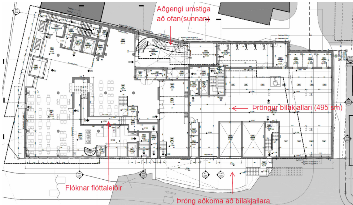
Mynd 5 - Jarðhæð
