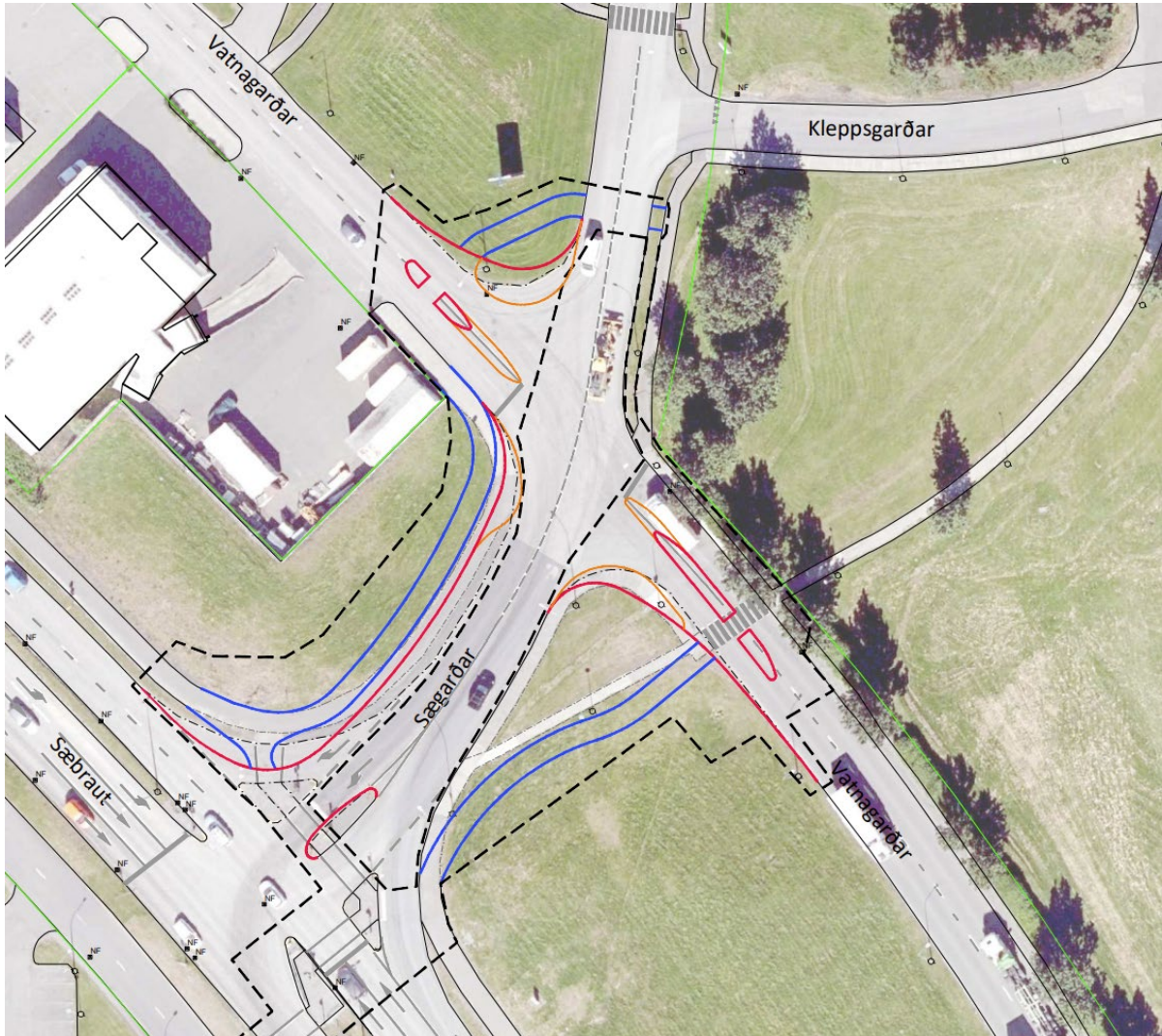
Mynd 1 Forhönnun að breytingum á gatnamótum Sægarða við Vatnagarða og við Sæbraut.
