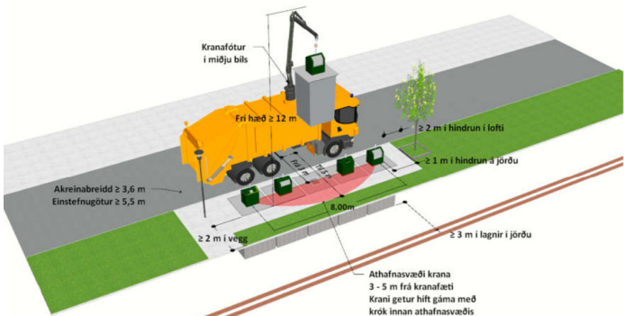
Mynd úr "Hönnunarviðmiðum um úrgangslausnir við íbúðarhúsnæði í Reykjavík". Nauðsynlegt rými umhverfis djúpgáma.
