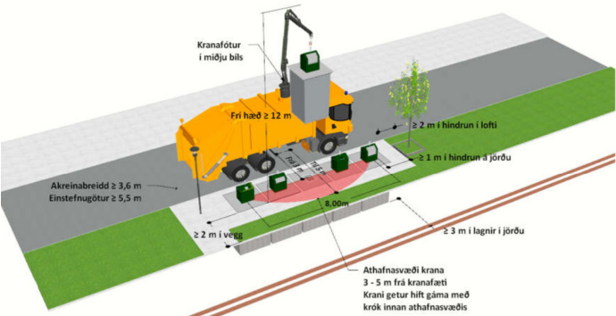
Mynd úr "Hönnunarviðmiðum um úrgangslausnir við íbúðarhúsnæði í Reykjavík". Nauðsynlegt rými umhverfis djúpgáma.
