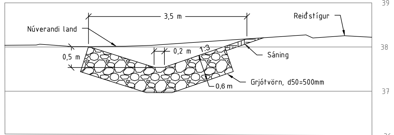
D SNID SKURÐUR 001 1:50
