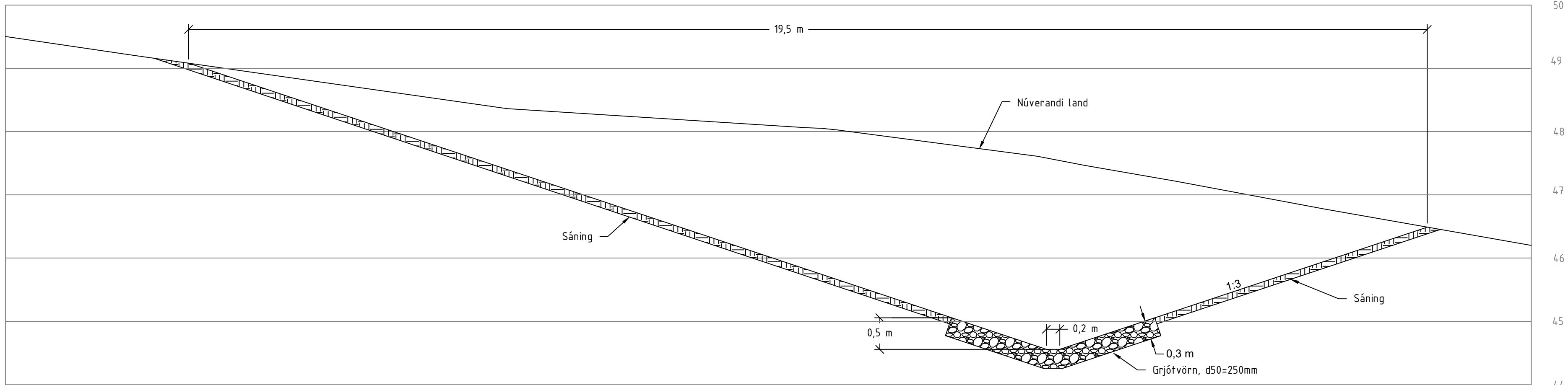
B SNID SKURÐUR 001 1:50
