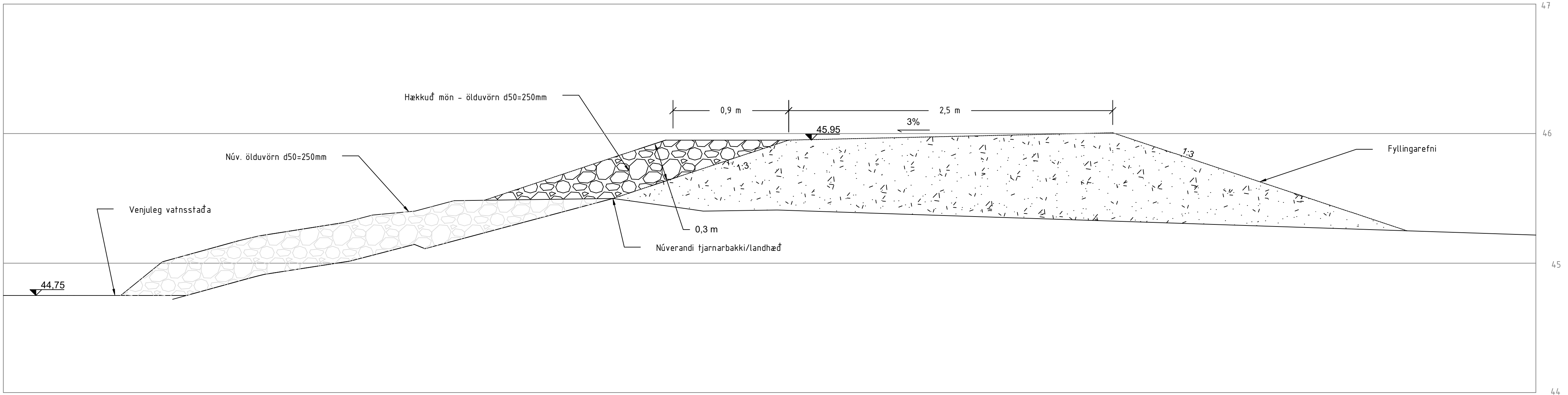
E SNID MÖN 001 1:20
