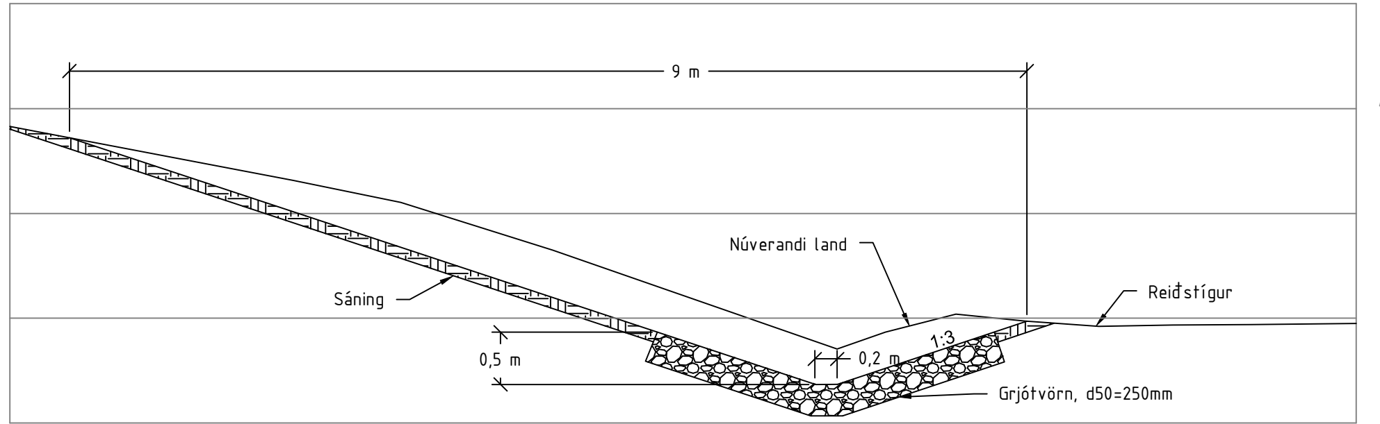
C SNID SKURÐUR 001 1:50
