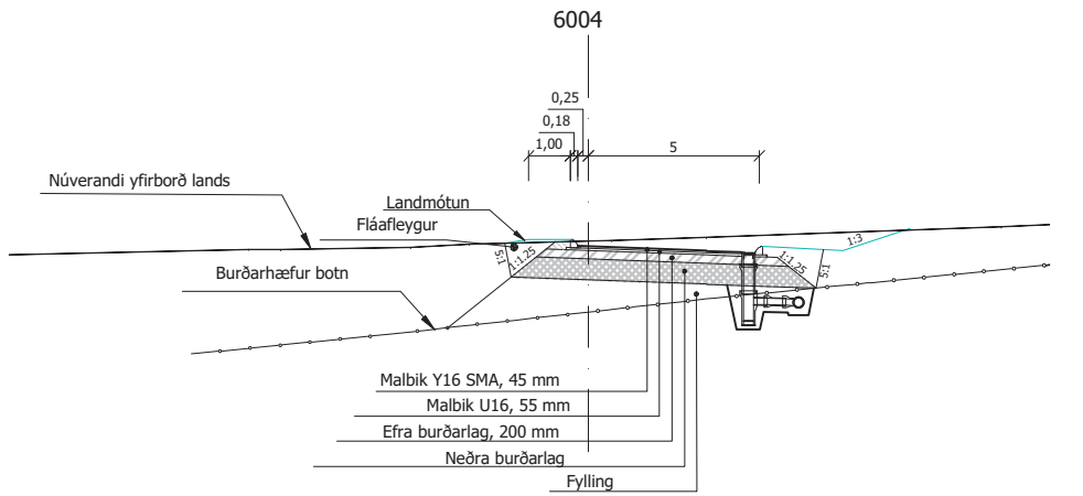
Kennisnið í rampa 6004 Mkv.: 1:100
