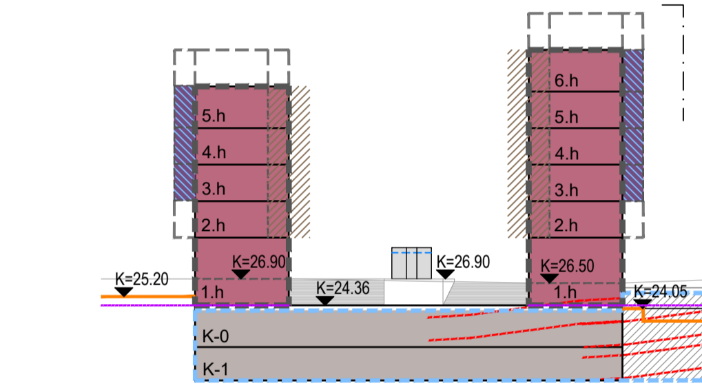
Sneiðing A-A
