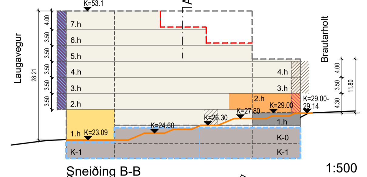
Sneiðing B-B 1:500
