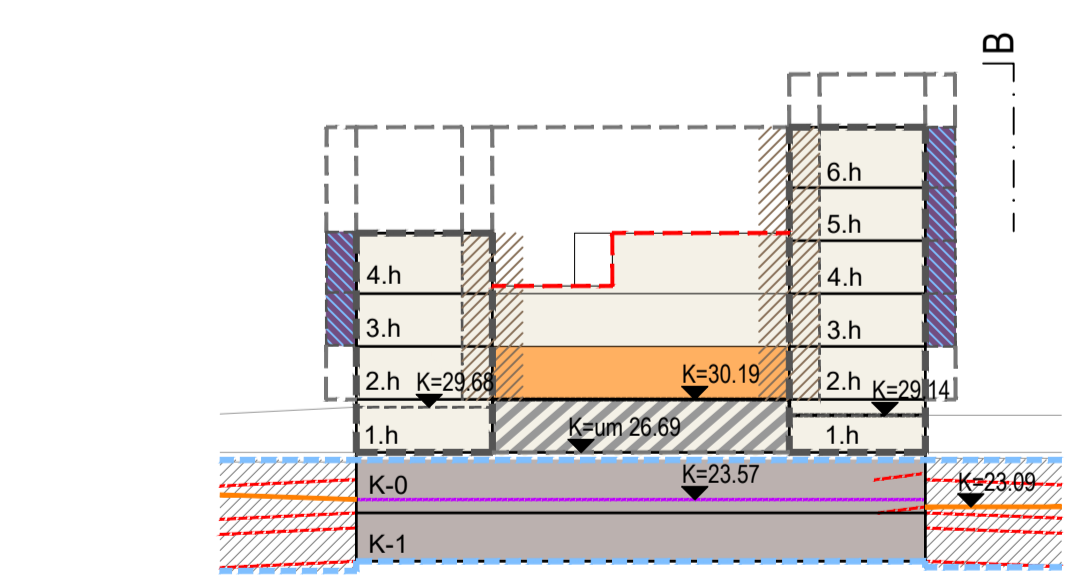
Sneiðing A-A
