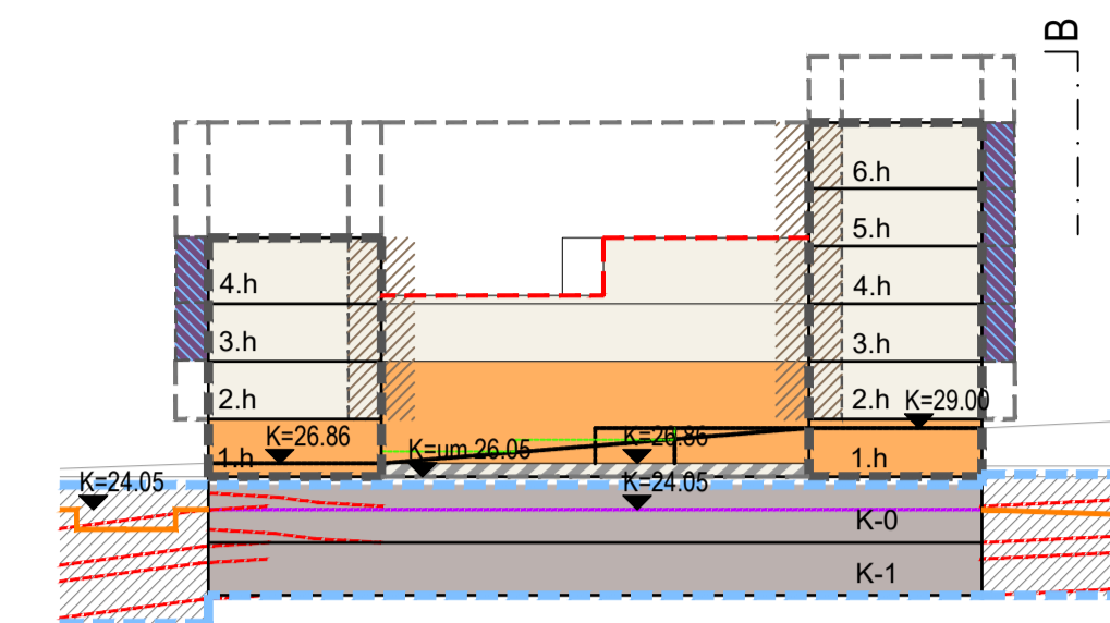
Sneiðing A-A
