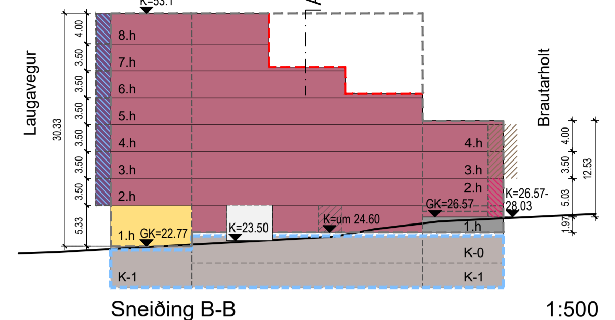
Sneiðing B-B 1:500
