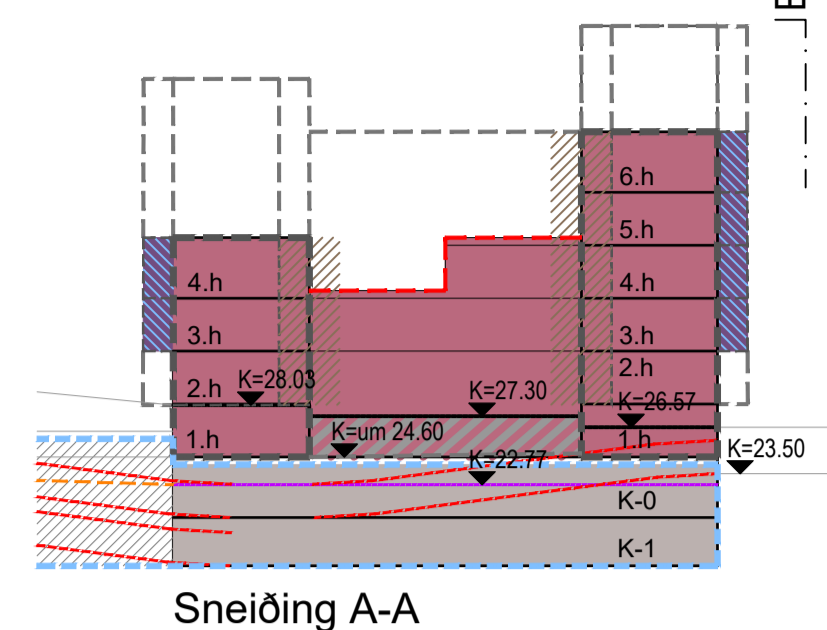
Sneiðing A-A
