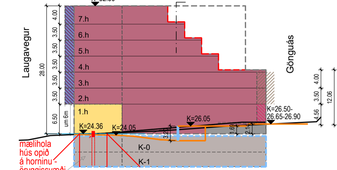
Sneiðing B-B
