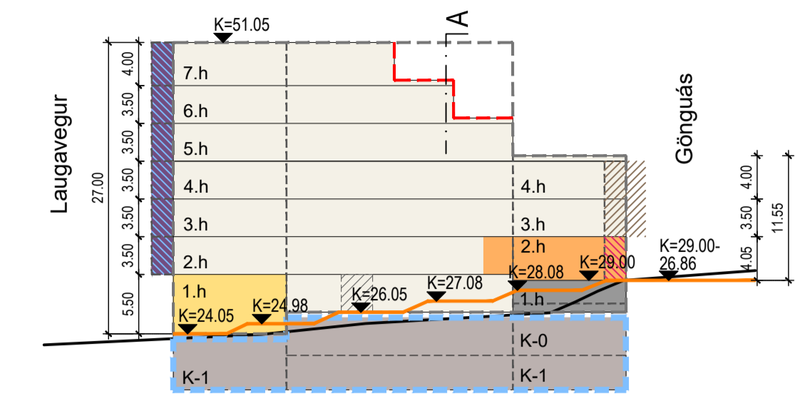
Sneiðing B-B
