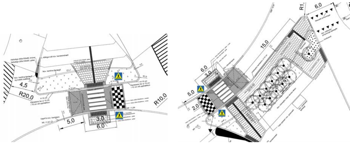
Mynd 2 Drög að útfærslu þrengingar og gangbrautar. Hægri – Við Melaskóla. Vinstri – Við Hótel Sögu.
