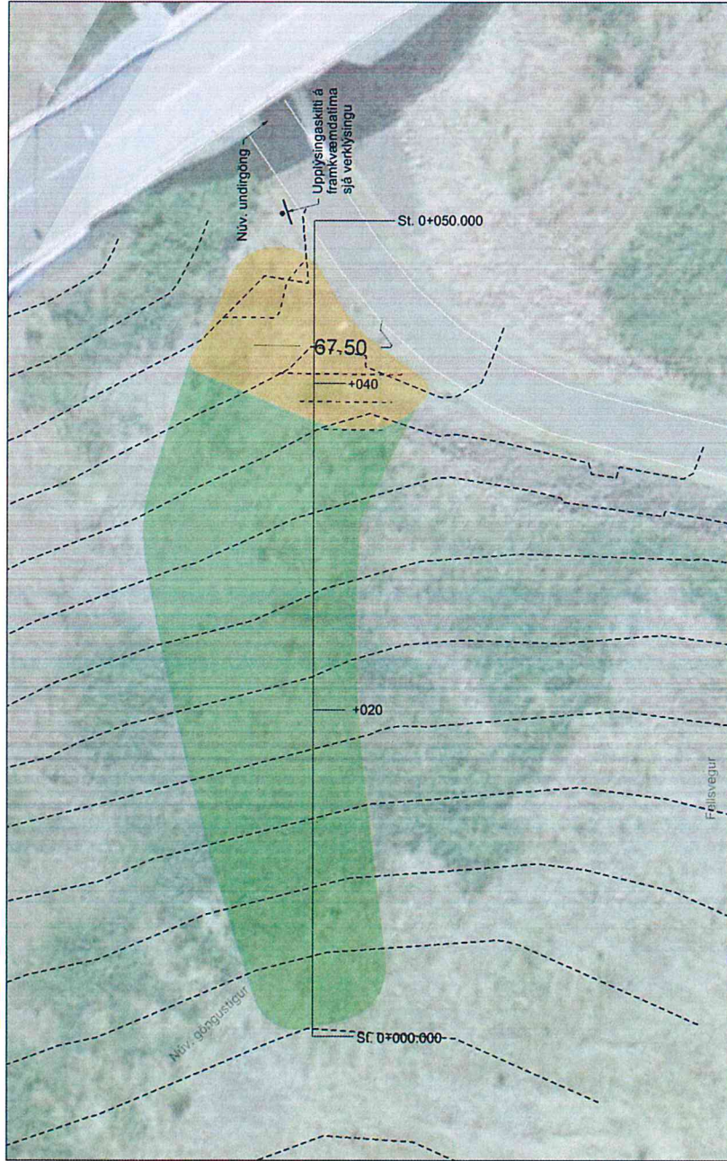
Reynisvatnsís sleobækka Grunnmynd 1:200
