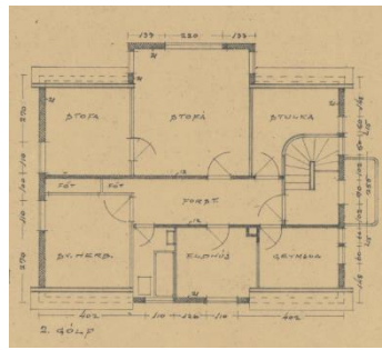
Samþykktar byggingarnefndateikningar af risibúð hússins.
