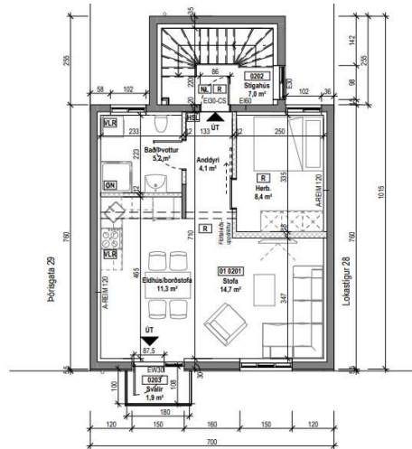
Grunnmynd af 2. hæð.
