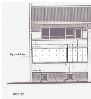
ÚTLIT SUÐUR 1:100
