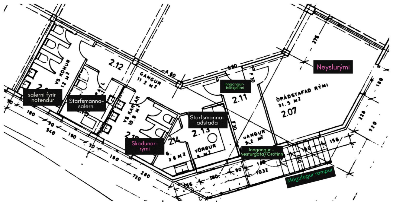
Drög að skoðunarrými skv. b-lið 7. gr. reglugerðar um neyslurými
