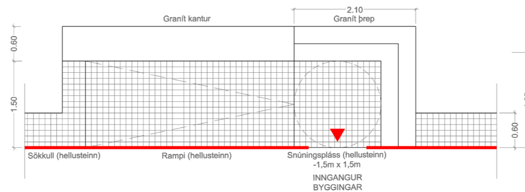
Týpólógía 3, þrjú þrep + skábraut - Grunnmynd
