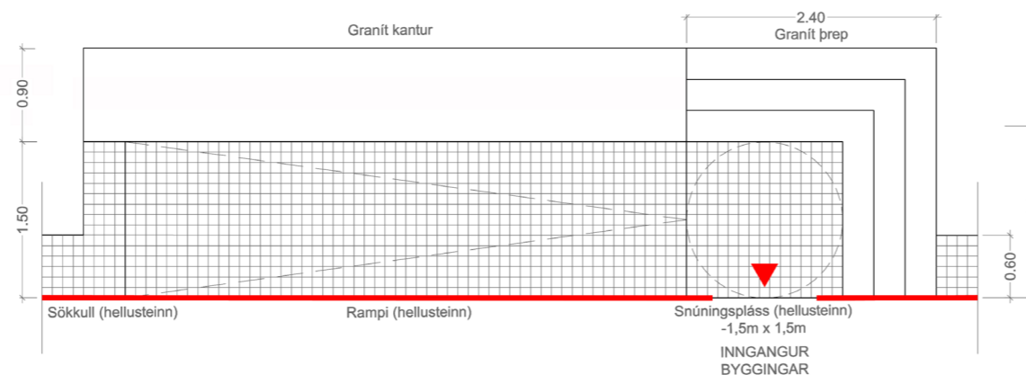
Týpólógía 3, þrjú þrep + skábraut - Grunnmynd
