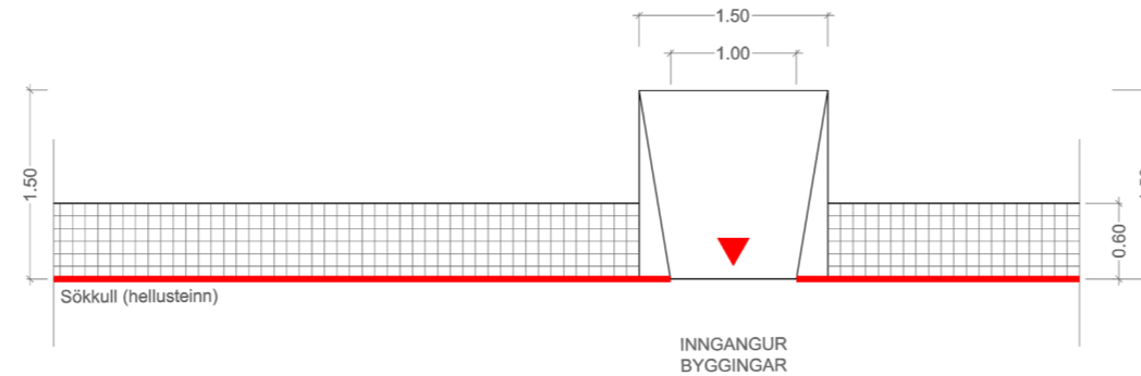
Týpólógía 2, tvö þrep + skábraut - Grunnmynd
