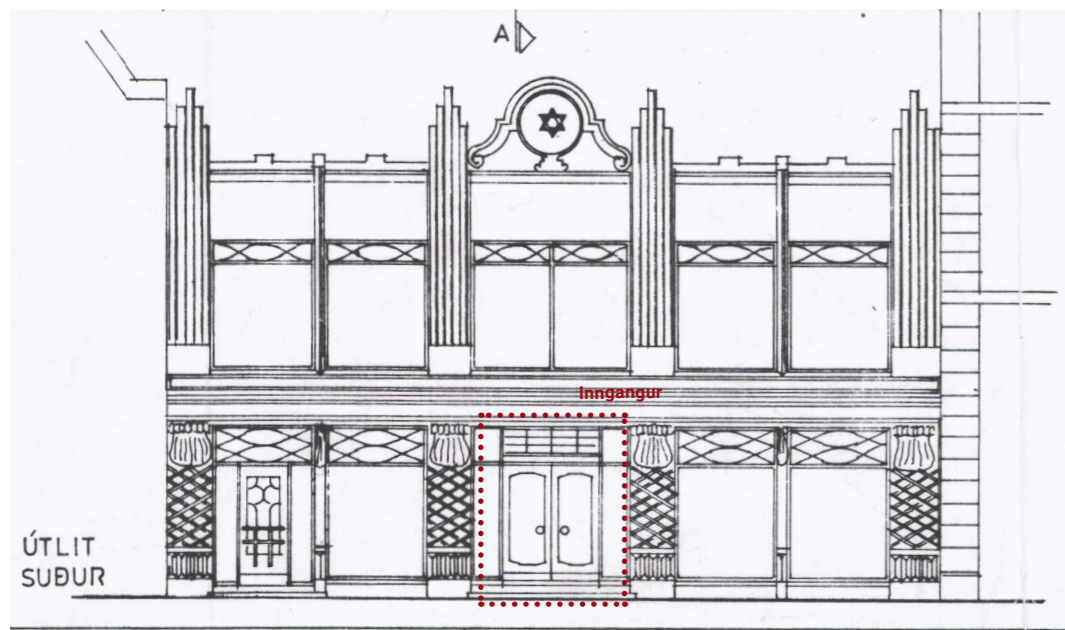
Aðaluppdráttur - Útlitstekning byggingar
