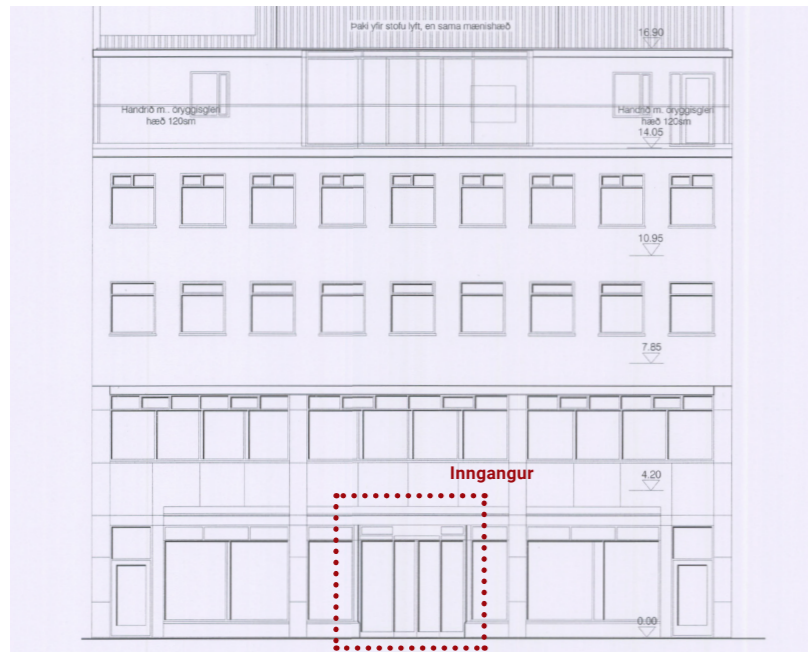
Aðaluppdráttur - Útlitsteikning byggingar
