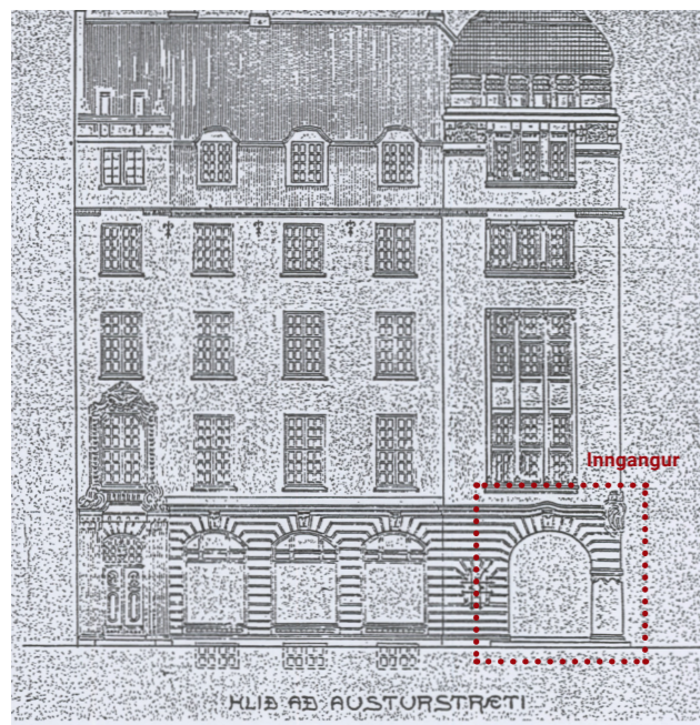
Aðaluppdráttur - Útlitstekning byggingar
