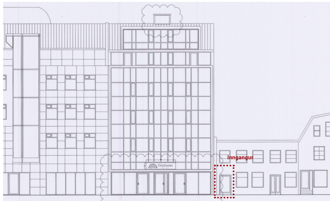
Aðaluppdráttur - Útlitsteikning byggingar
