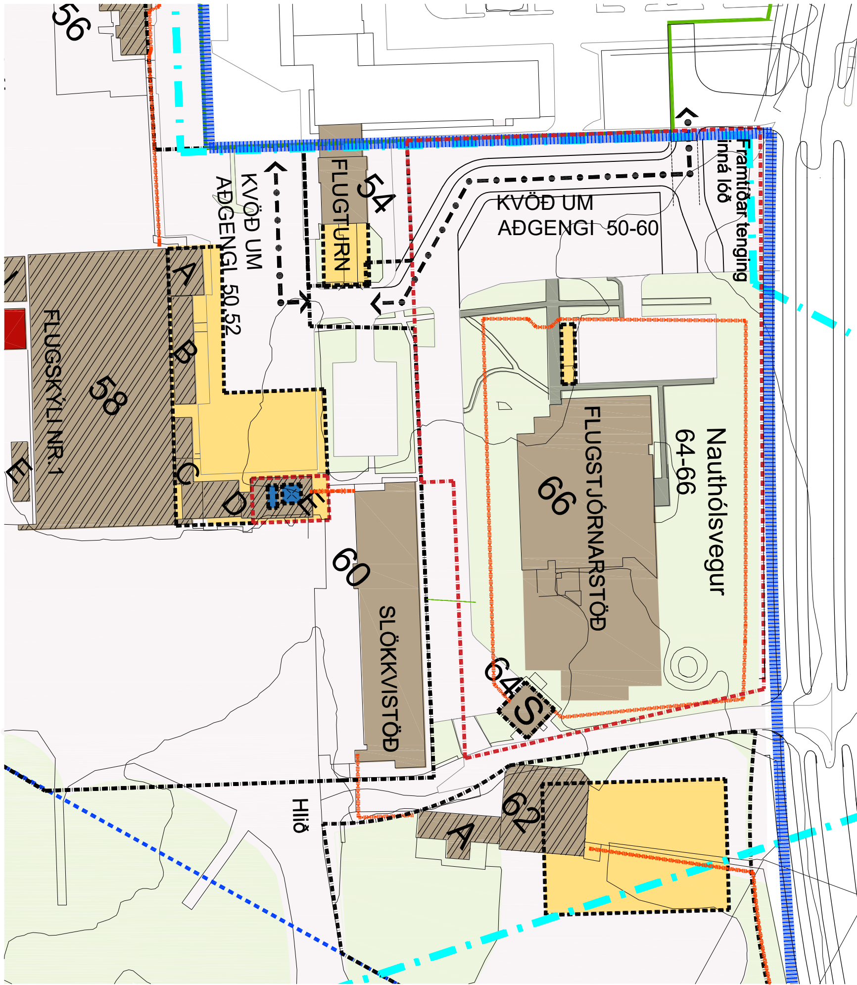
TILLAGA AÐ DEILISKIPULAG REYKJAVÍKURFLUGVALLAR, mkv. 1:1000
