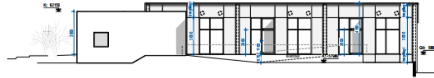
6 ÚTLIT - SUÐUR / GARDHLÍÐ - eftir breytingu M 1:100
