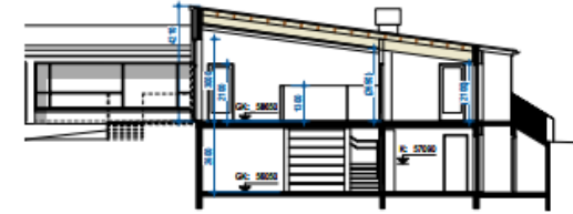
5 SNEIÐING D-D M 1:100
