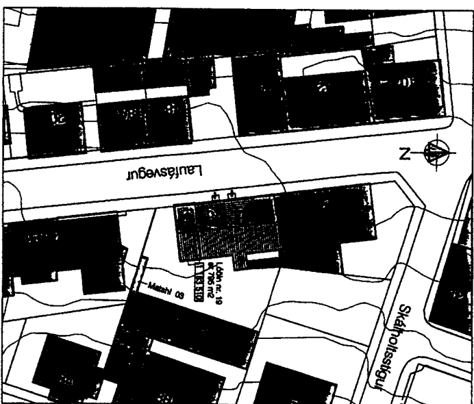
Afstöðumynd 1:500
