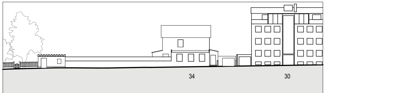
C - C | Útlit Þingholtsstræti 1:500 m.v. A1
