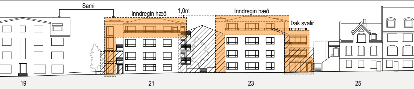
D - D | Útlit Laufásvegur 1:500 m.v. A1
