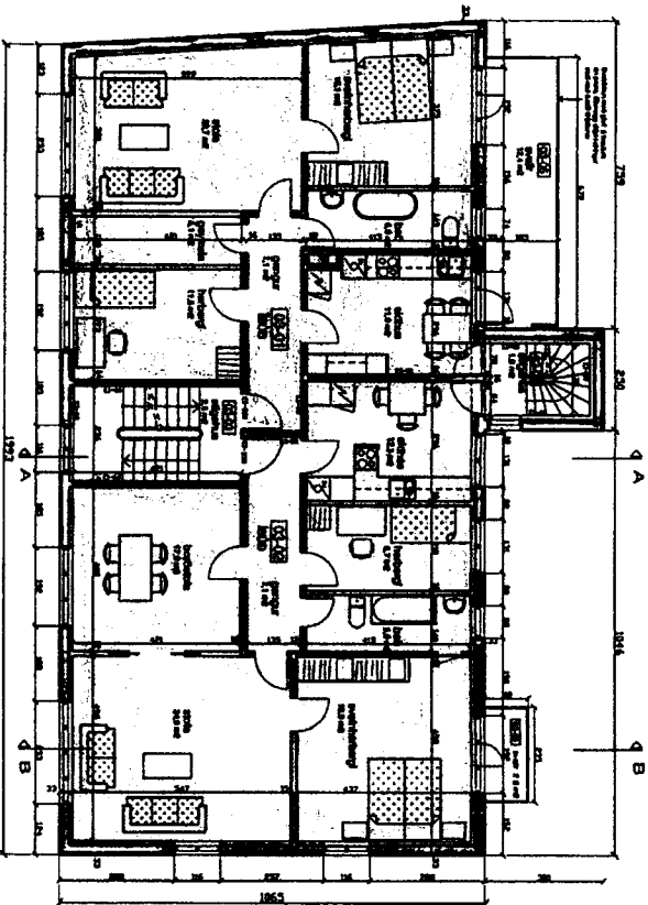
grunnmynd 3.hæðar
