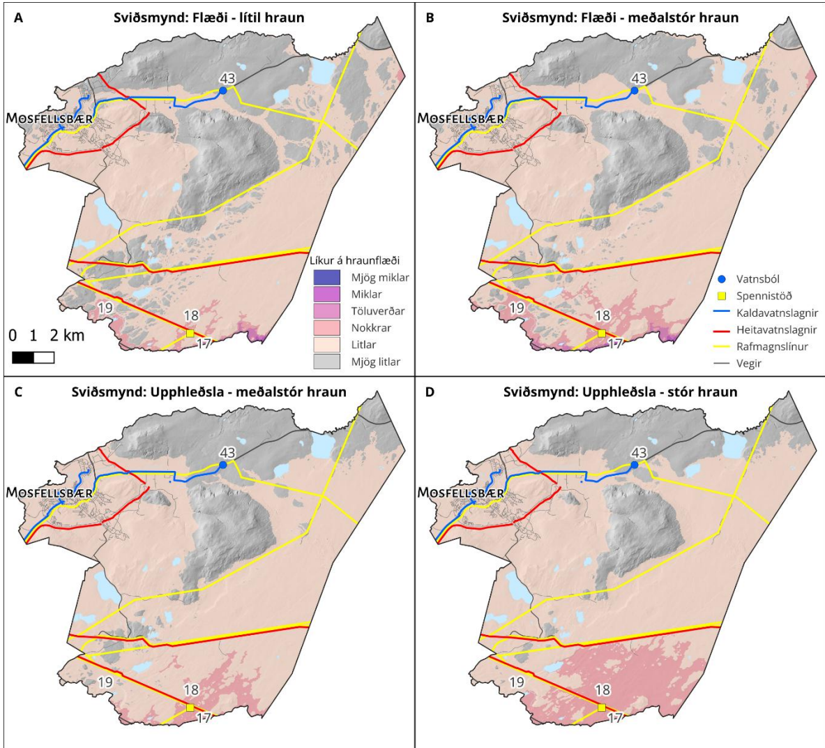
Mynd 15. Líkur á hraunflæði innan sveitarfélagsins Mosfellsbæjar skv. niðurstöðum sviðsmýndanna fjögurra (sjá kafla 2.2) og að teknu tilliti til vægis hermigosupptaka. Efri myndirnar tvær sýna niðurstöður miðað við hermanir sem gerðar eru með Flæðistillingu (lítill hraun: V=0,02 \text{ km}^3 ; meðalstór hraun V=0,1 \text{ km}^3 ) en neðri myndirnar með Upphleðslustillingu (meðalstór hraun: V=0,1 \text{ km}^3 ; stór hraun V=0,3 \text{ km}^3 ). Sviðsmýndin Upphleðsla – stór hraun ógnar stærsta svæðinu og sýnir mestar líkur á hraunflæði. Dekkri litir tákna meiri líkur og þ.a.l. svæði sem eru berskjaldaðri fyrir hraunflæði. Á myndunum eru sýndar helstu raflínur, vatnslagnir (heitt og kalt vatn) og vegir.
