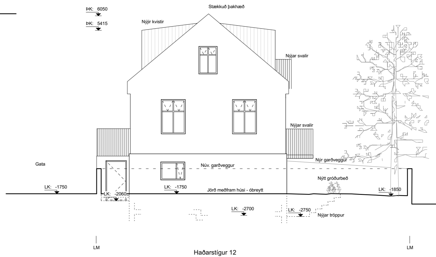
Ásýnd suðvestur mkv: 1:100
