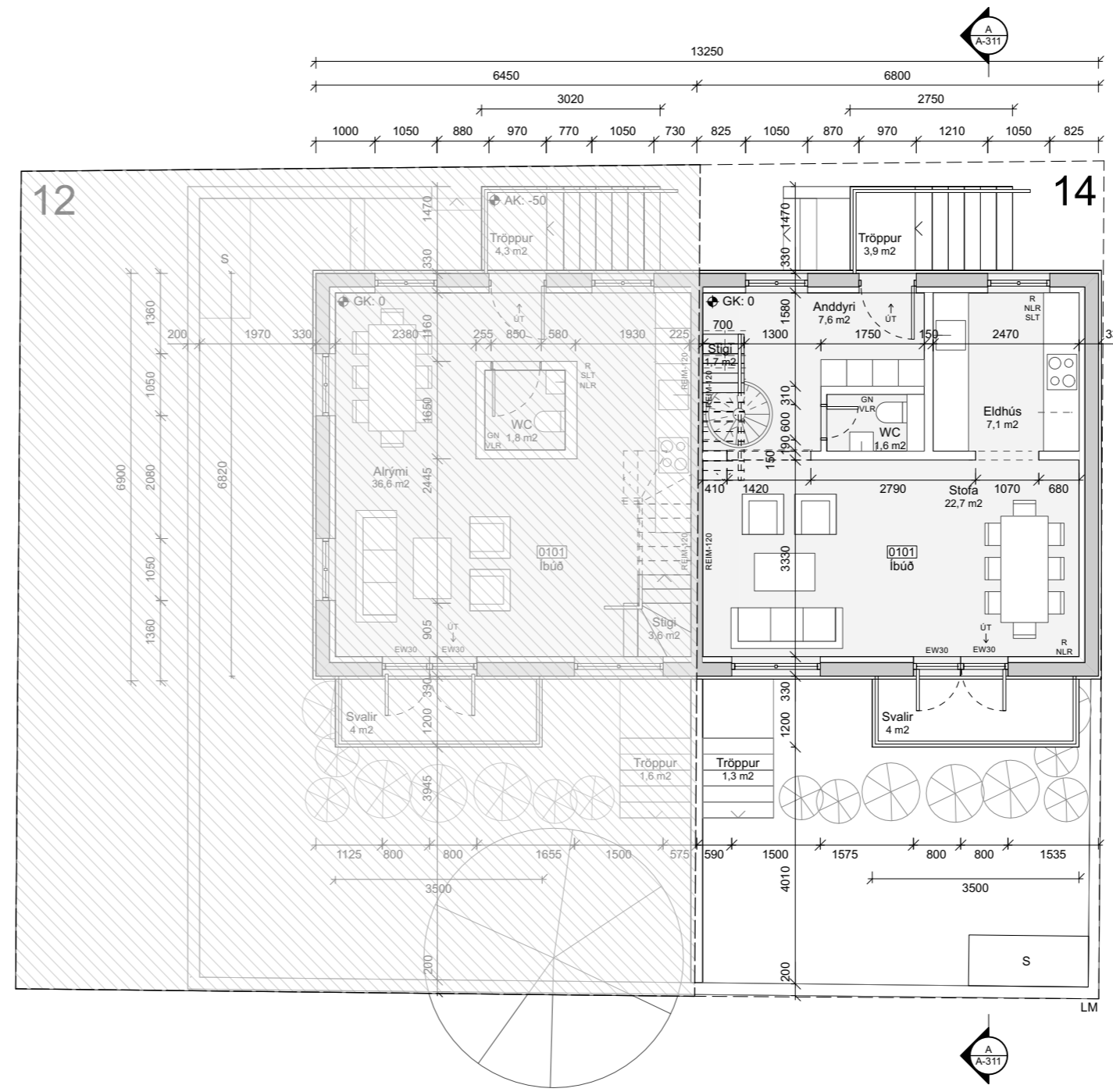
Grunnmynd 1. hæðar Mkv: 1:100
