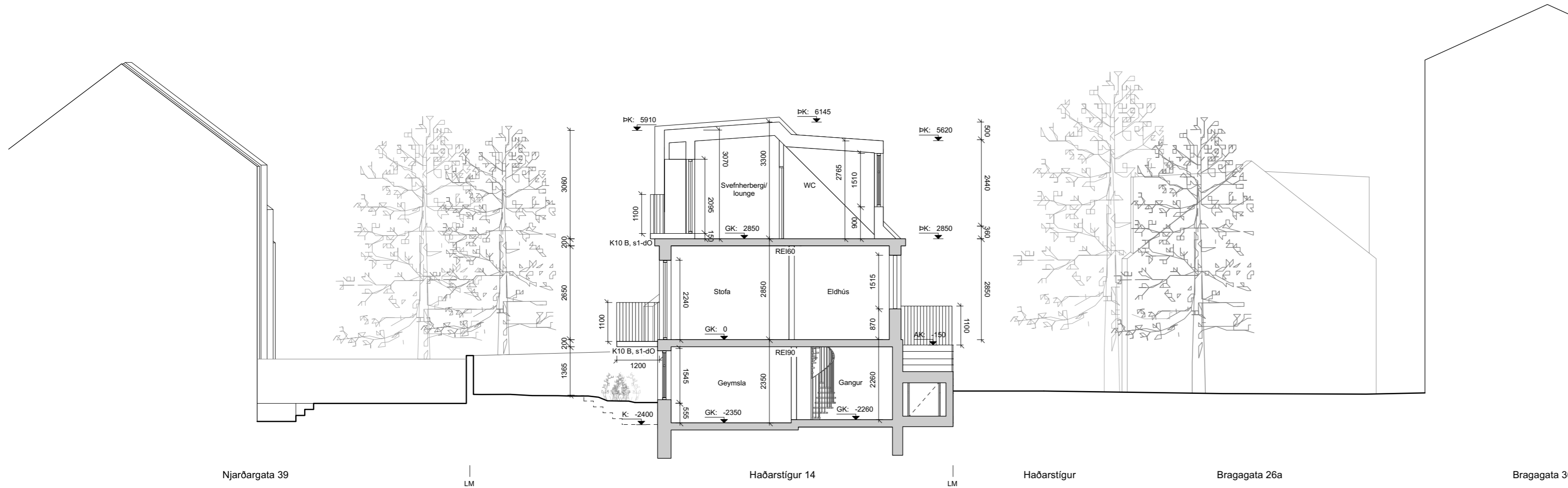
Sníð A-A Mkv: 1:100
