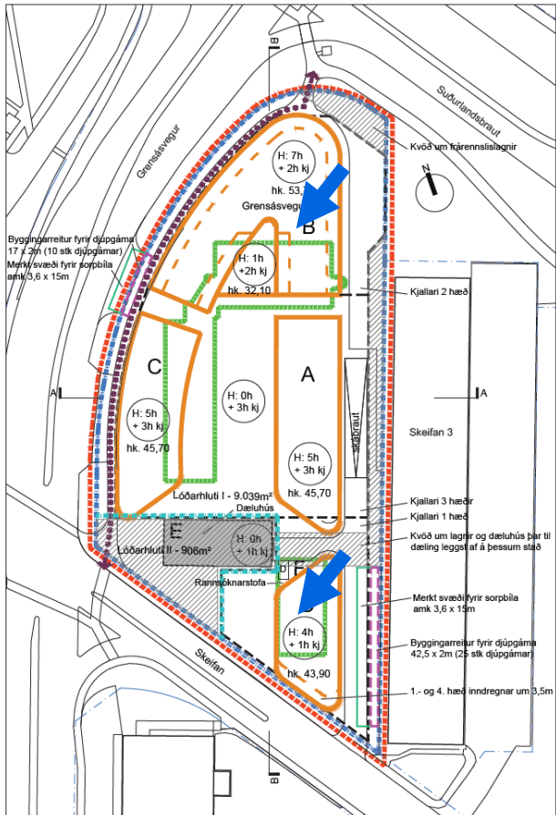
Gildandi deiliskipulag samþykkt 26.01.2023, auglýst í B-deild stjórnartíðinda 13.02.2023. MKV 1:1000
