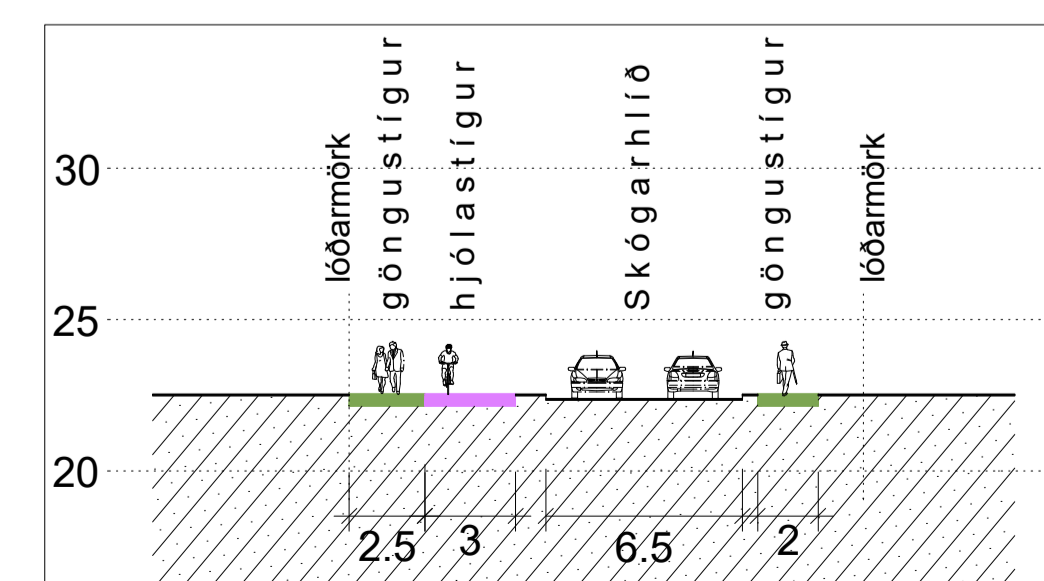
Sneiðing A - A M 1:250 Sneiðing í Skógarhlíð
