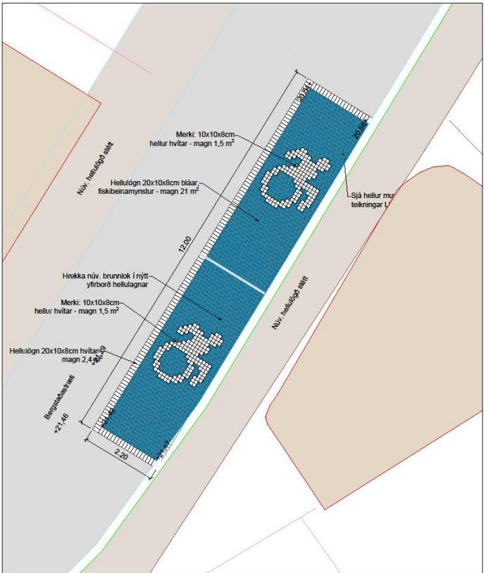
Grunnmynd, mælikvarði 1:50
