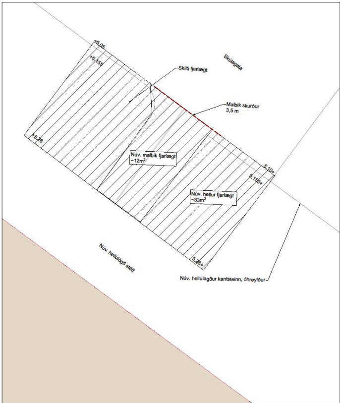
Upprifsmynd, mæliskvarði 1:50
