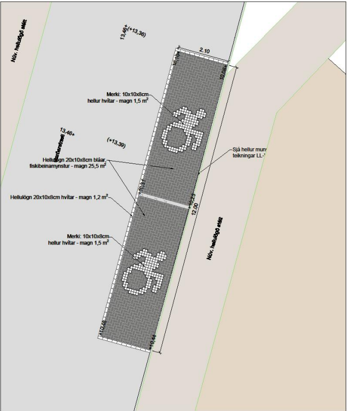
Grunnmynd, mælikvarði 1:50
