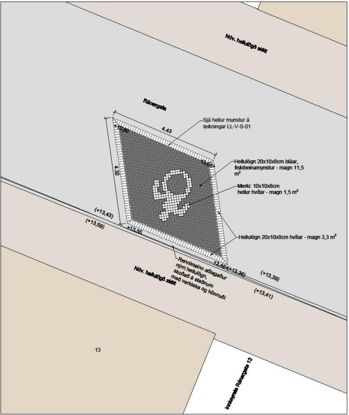
Grunnmynd, mælikvarði 1:50
