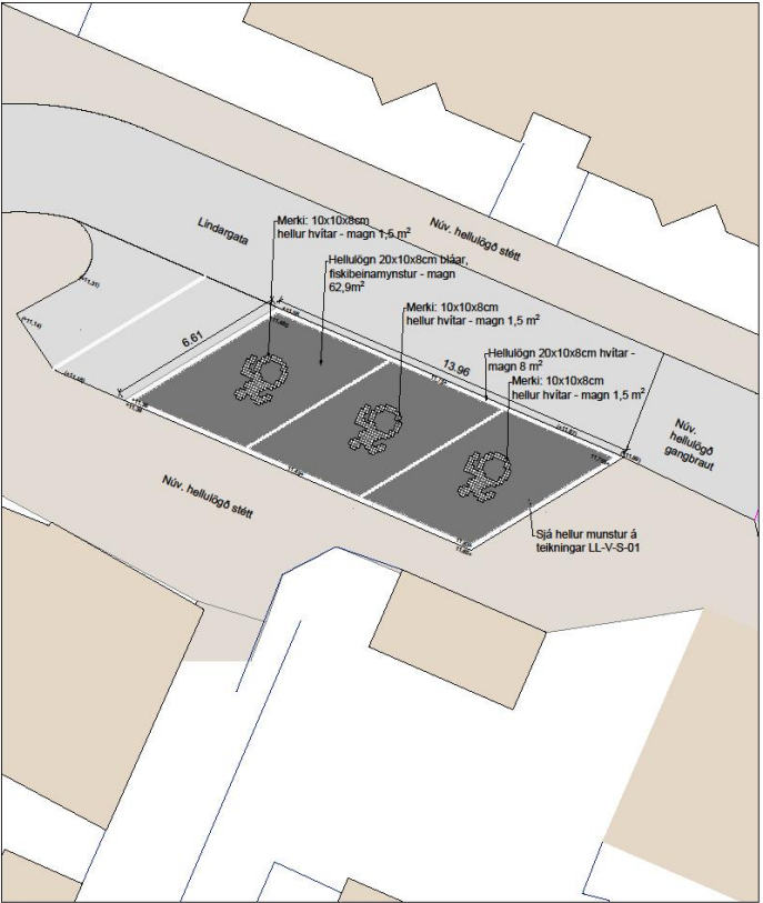
Grunnmynd, mæliskvarði 1:100
