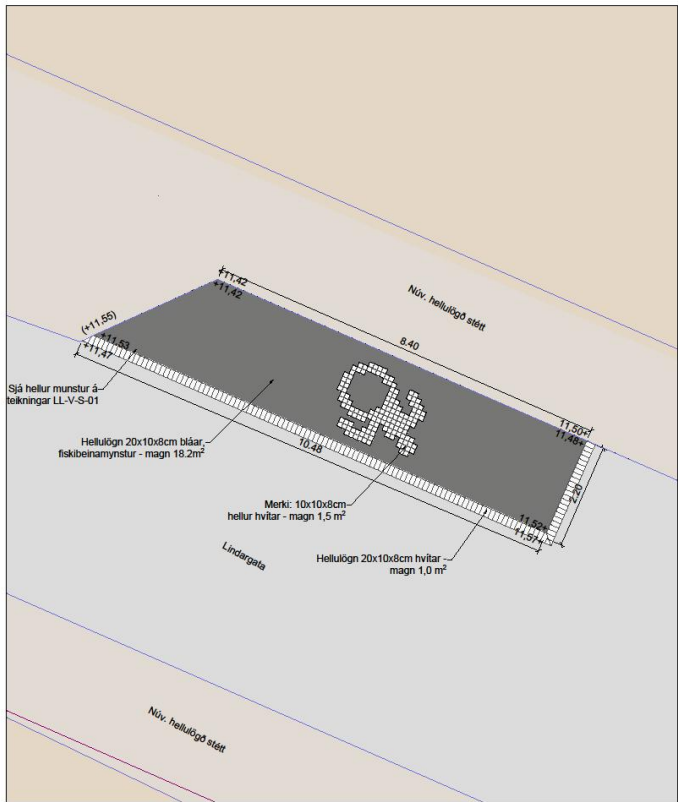
Grunnmynd, mælikvarði 1:50
