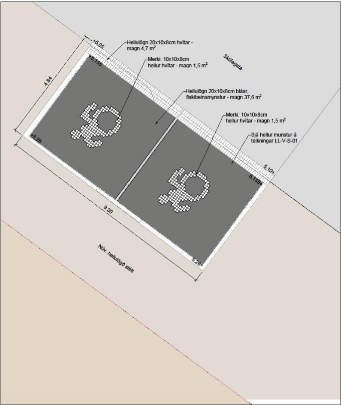
Grunnmynd, mæliskvarði 1:50
