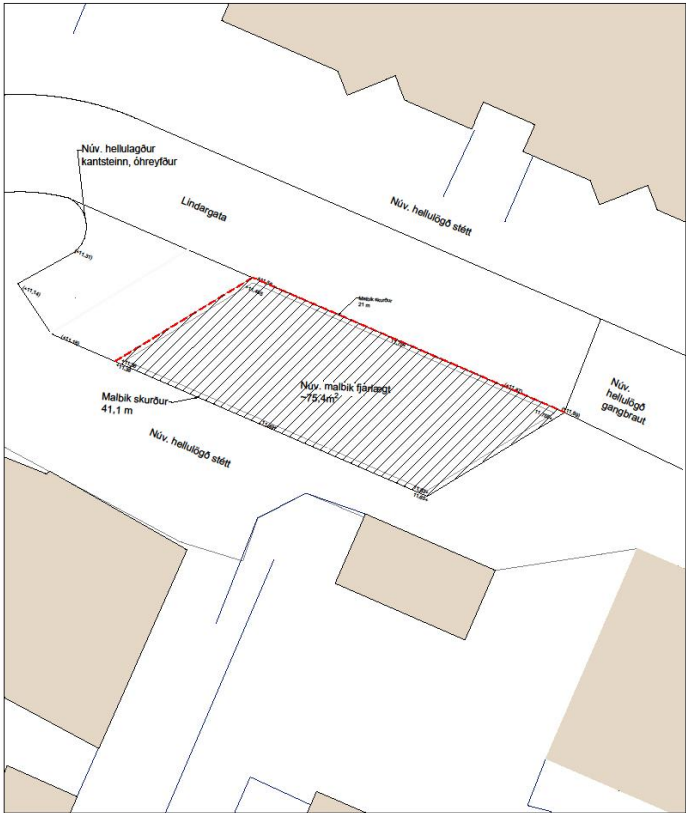
Upprifsmynd, mæliskvarði 1:100
