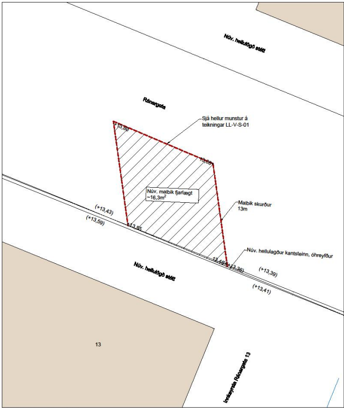
Upprifsmynd, mælikvarði 1:50
