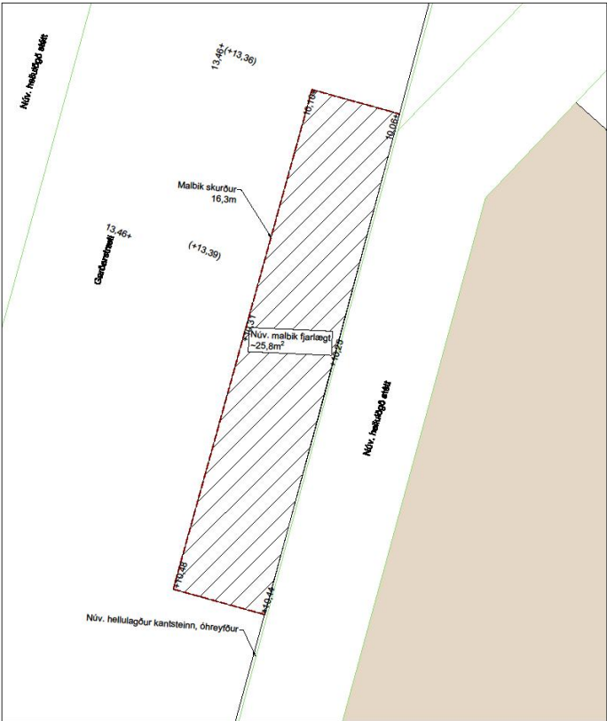
Upprifsmynd, mælikvarði 1:50
