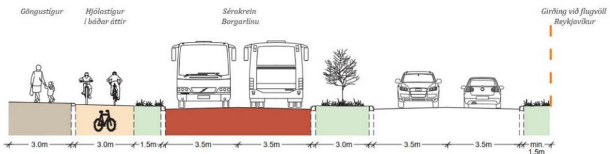
Mynd 1 Dæmi um þversnið af göturými Borgarlínunnar eftir framkvæmdir (úr umhverfismatsskýrslu)
