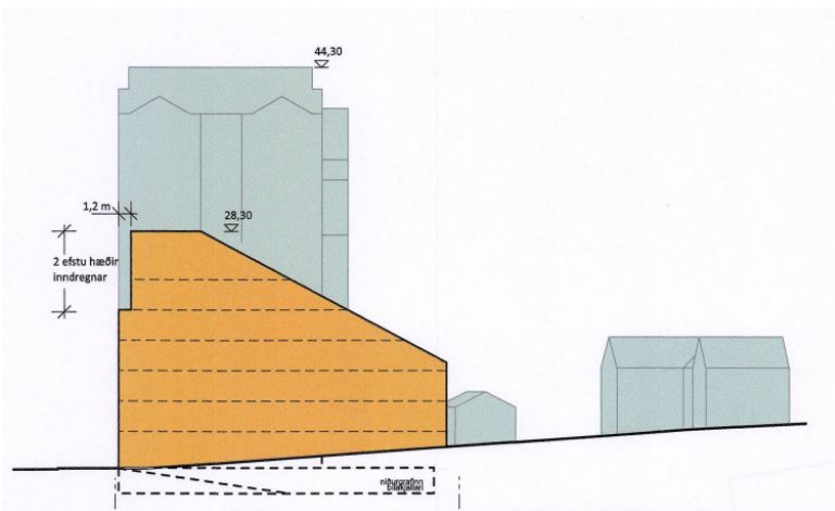
Snið AA
