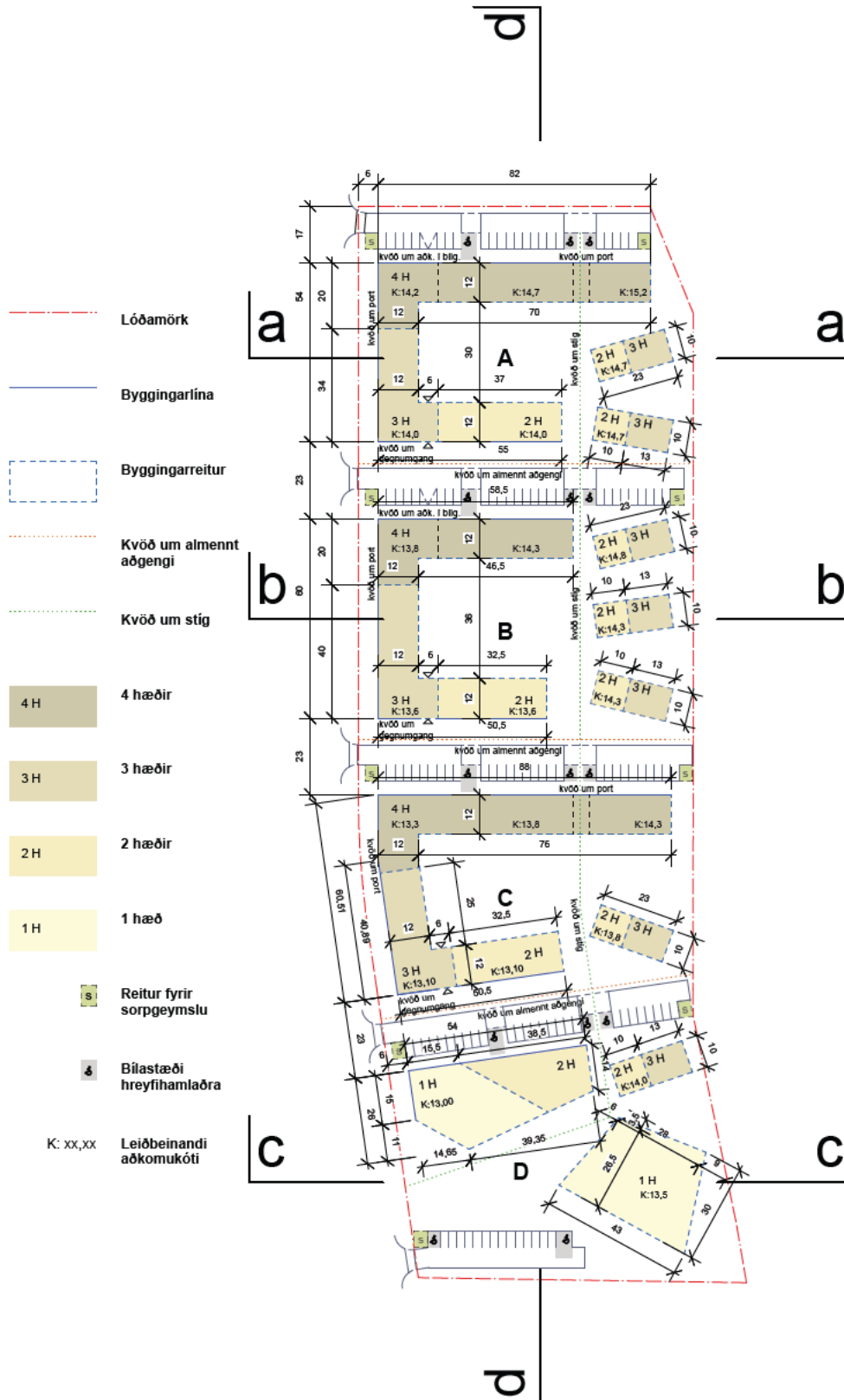
Mynd 23 Skilmálateikning.
