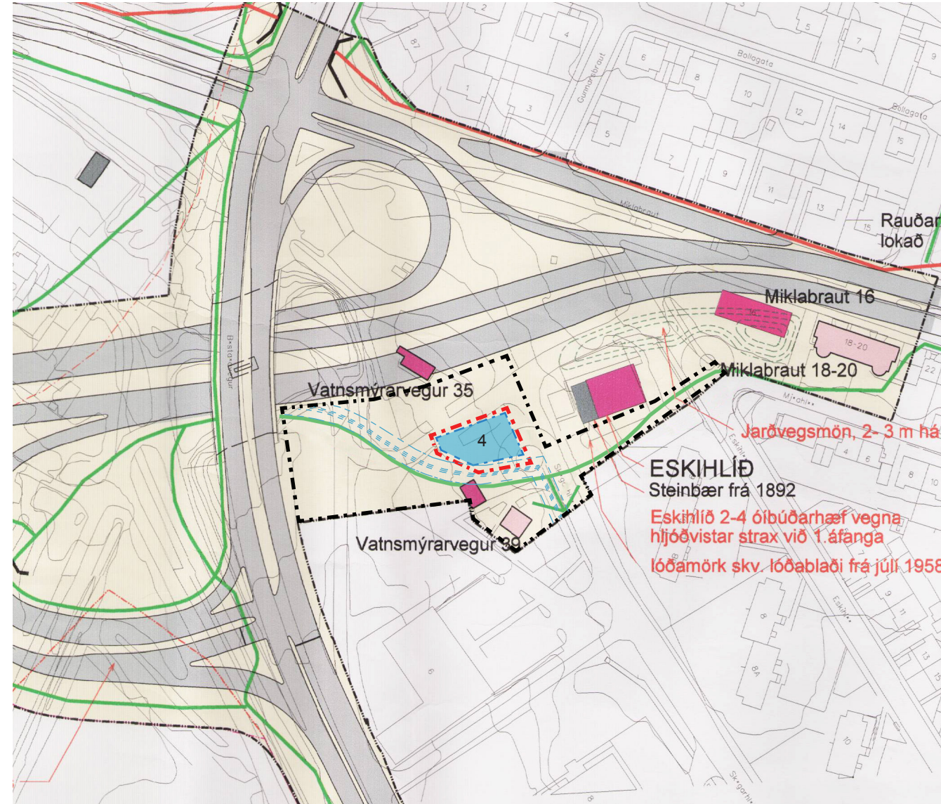
DEILISKIPULAGSBREYTING 1:2000
