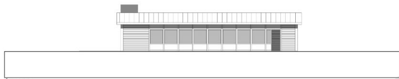
Útlit suður
