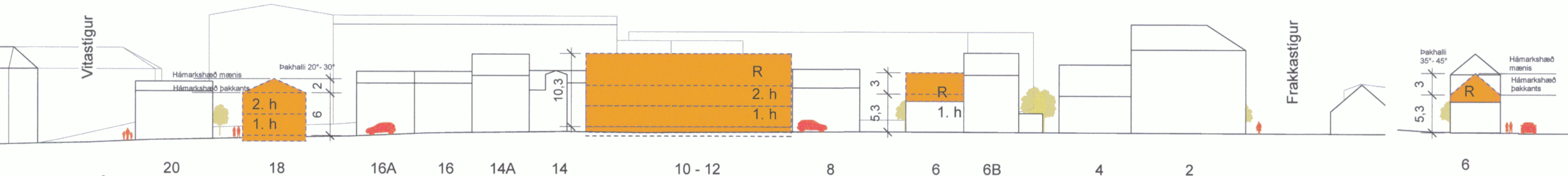
Snið 1-1 Ásýnd Bergþórugata, mkv. 1:500
