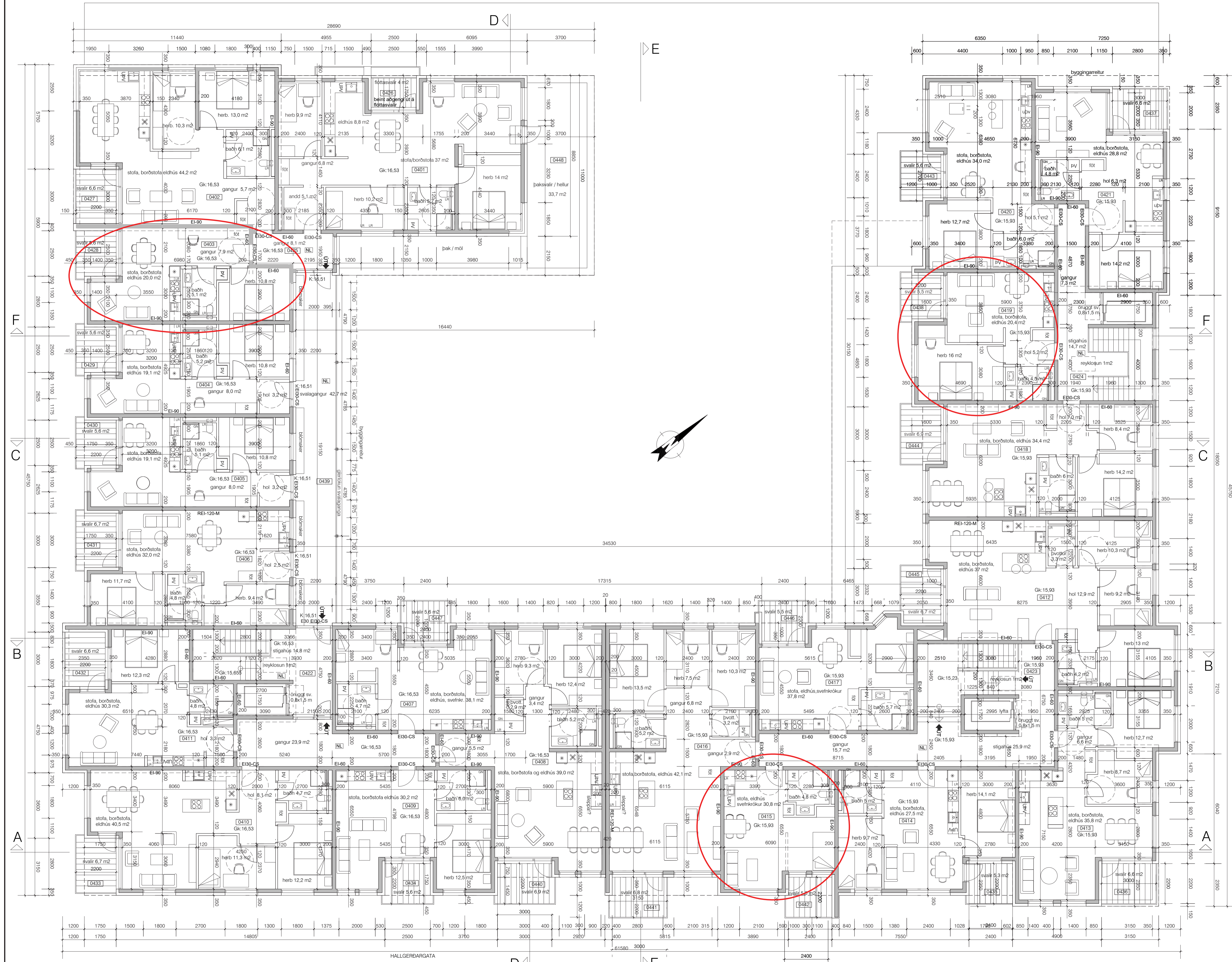
GRUNNMYND 4. HÆÐAR 21 íbúð
