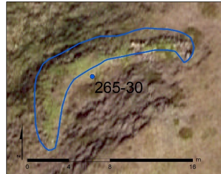
Mynd 19. Skotgröf (265-30) á nýlegri loftmynd, teiknað eftir uppmælingu.
