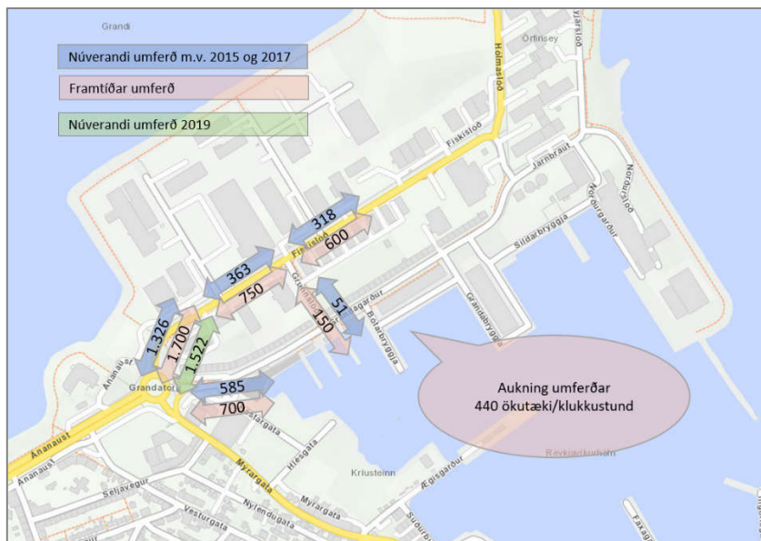
MYND 11 Væntanleg dreifing umferðar um skipulagssvæðið m.v. sviðsmynd 2. Umferð er áætluð m.v. fullbyggðan Línbergsgreit, ökut./klukkustund.
