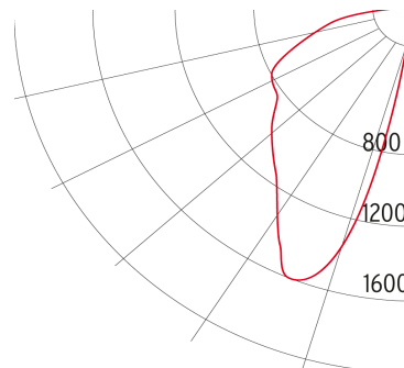
Dæmigerð ljósdreifing
