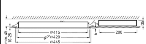
Dæmigerð ljósdreifing
