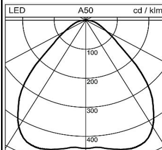
Dæmigerð stærð
