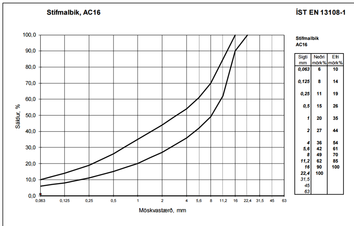
MYND 1 Stífmálbik, SL16
