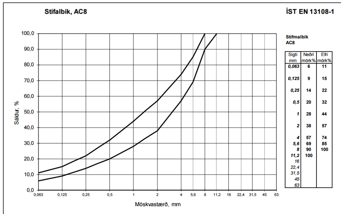
MYND 3 Stífbalbik, SL8
