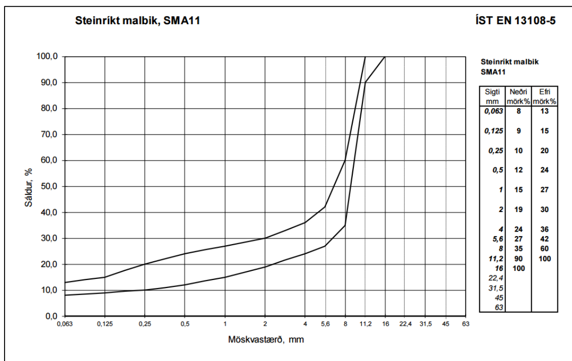
MYND 5 Steinríkt malbik, SMA11
