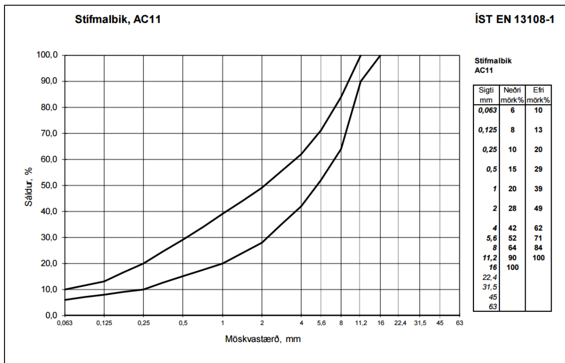
MYND 2 Stífmálbik, SL11
