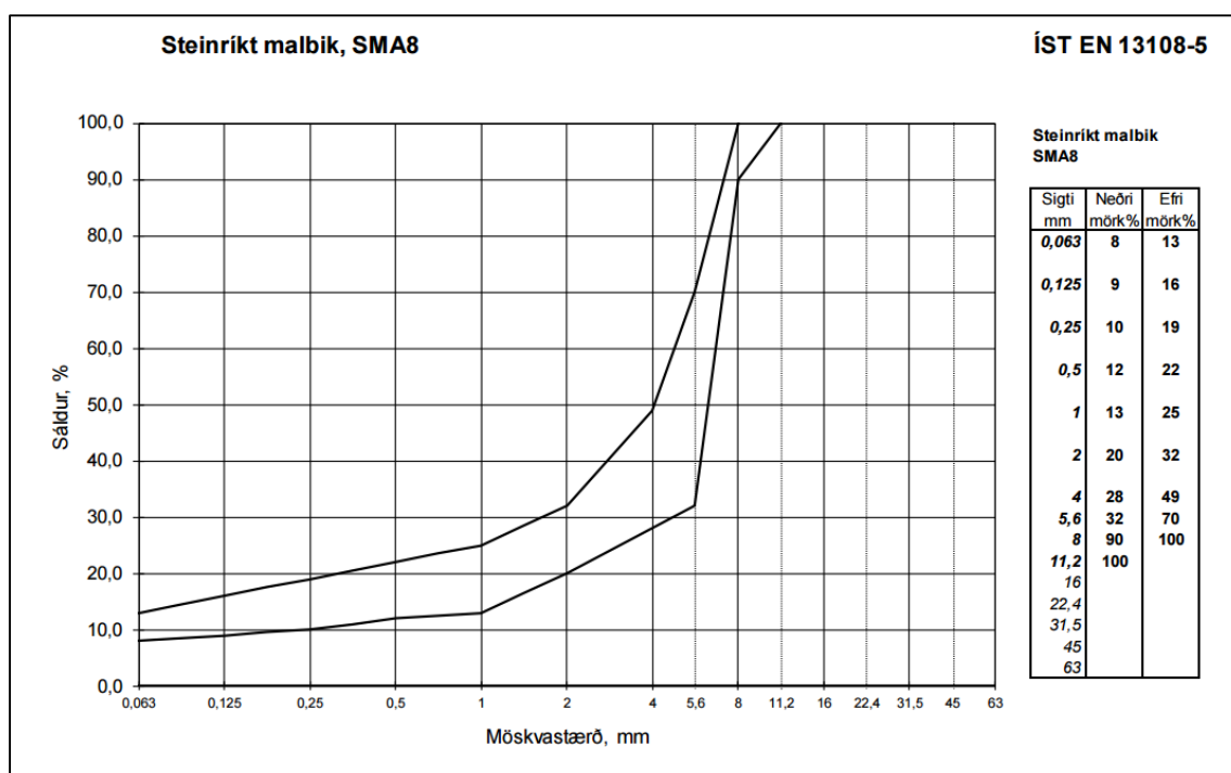
MYND 6 Steinríkt malbik, SMA8
