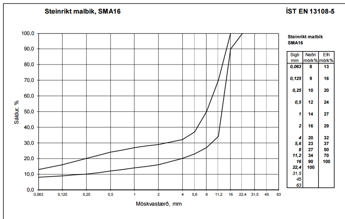
MYND 4 Steinríkt malbik, SMA16
