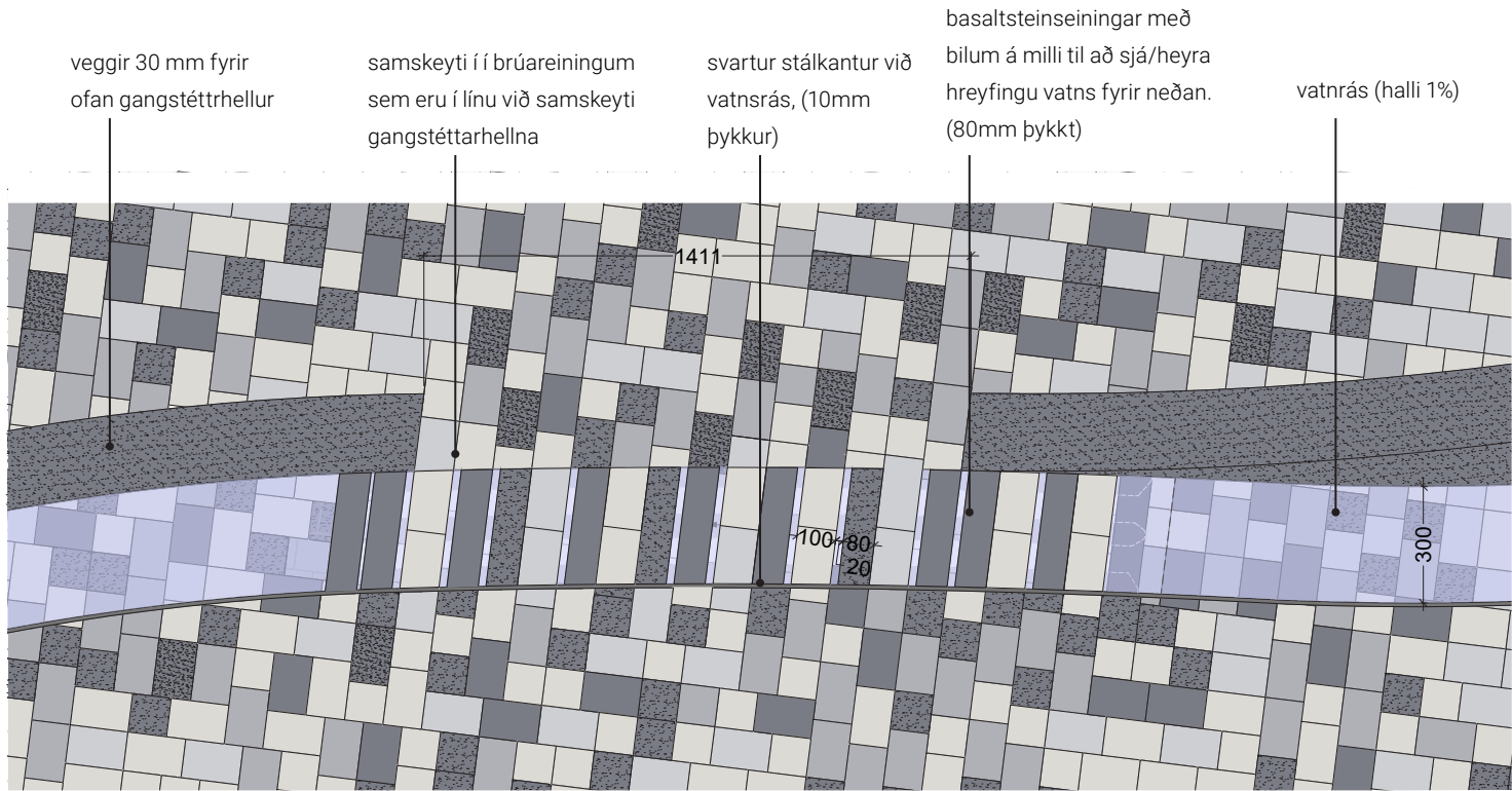
Brú yfir vatnsrás - skornar basaltseinseiningar lagðar sem framhald af gangstéttarhellum mælikvarði 1:200
