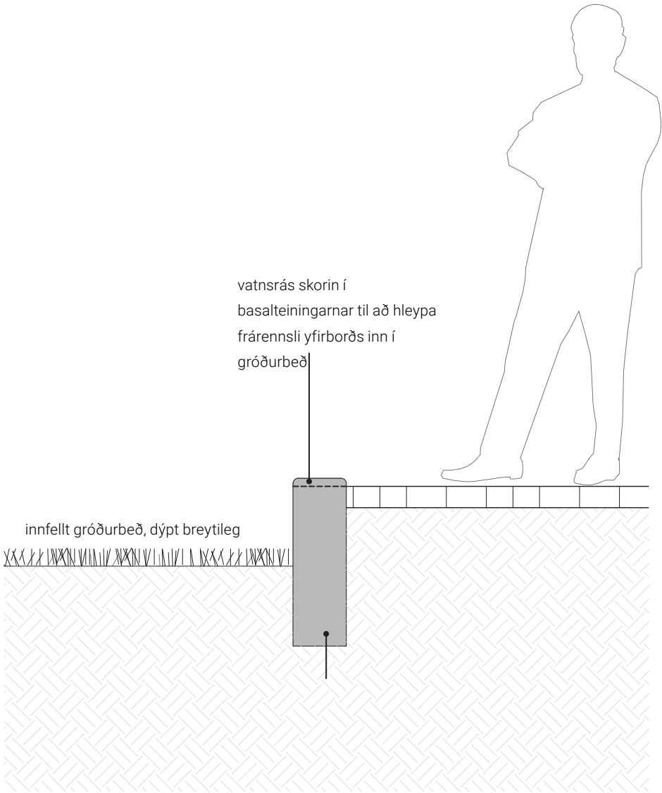
VEGGIR 2 - 7 200mm breiður stoðveggur með vatnsrás skorið í blokkeiningar
