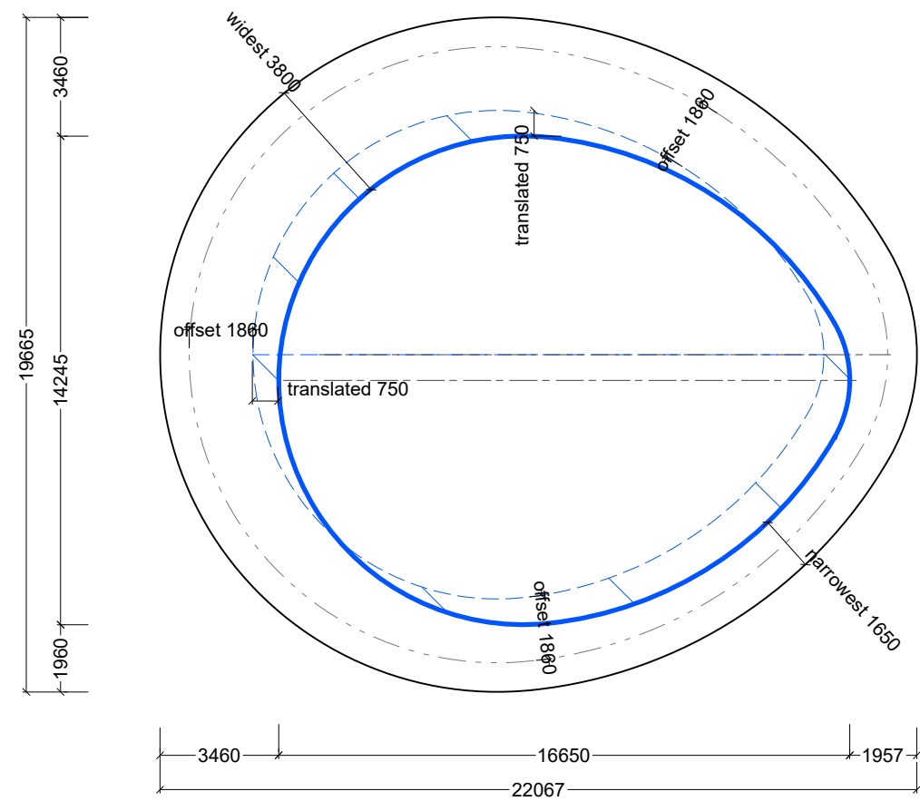
Innra form baugs (ens. oculus)
