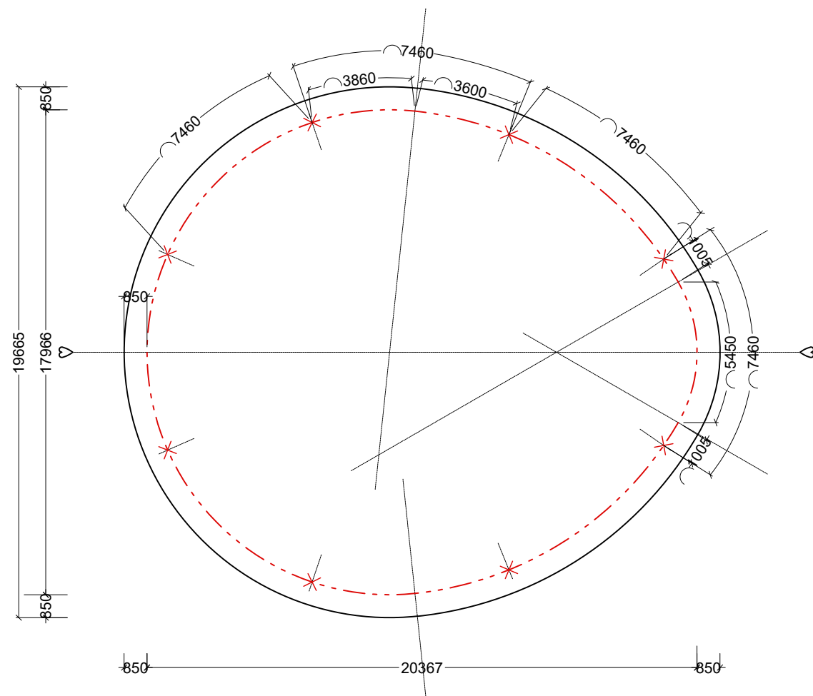
Ás burðarsúlur staðsett fyrir innan Bauginn
