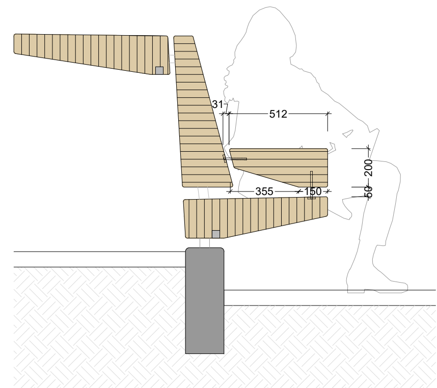
SNÍÐ B-B' Bekkur með armstoðir
