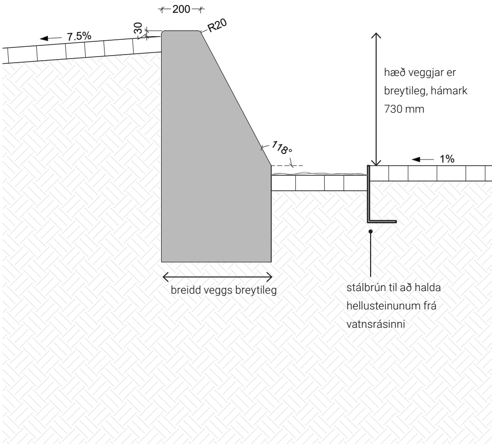
SNID B-B' Veggur á hæsta punkti
