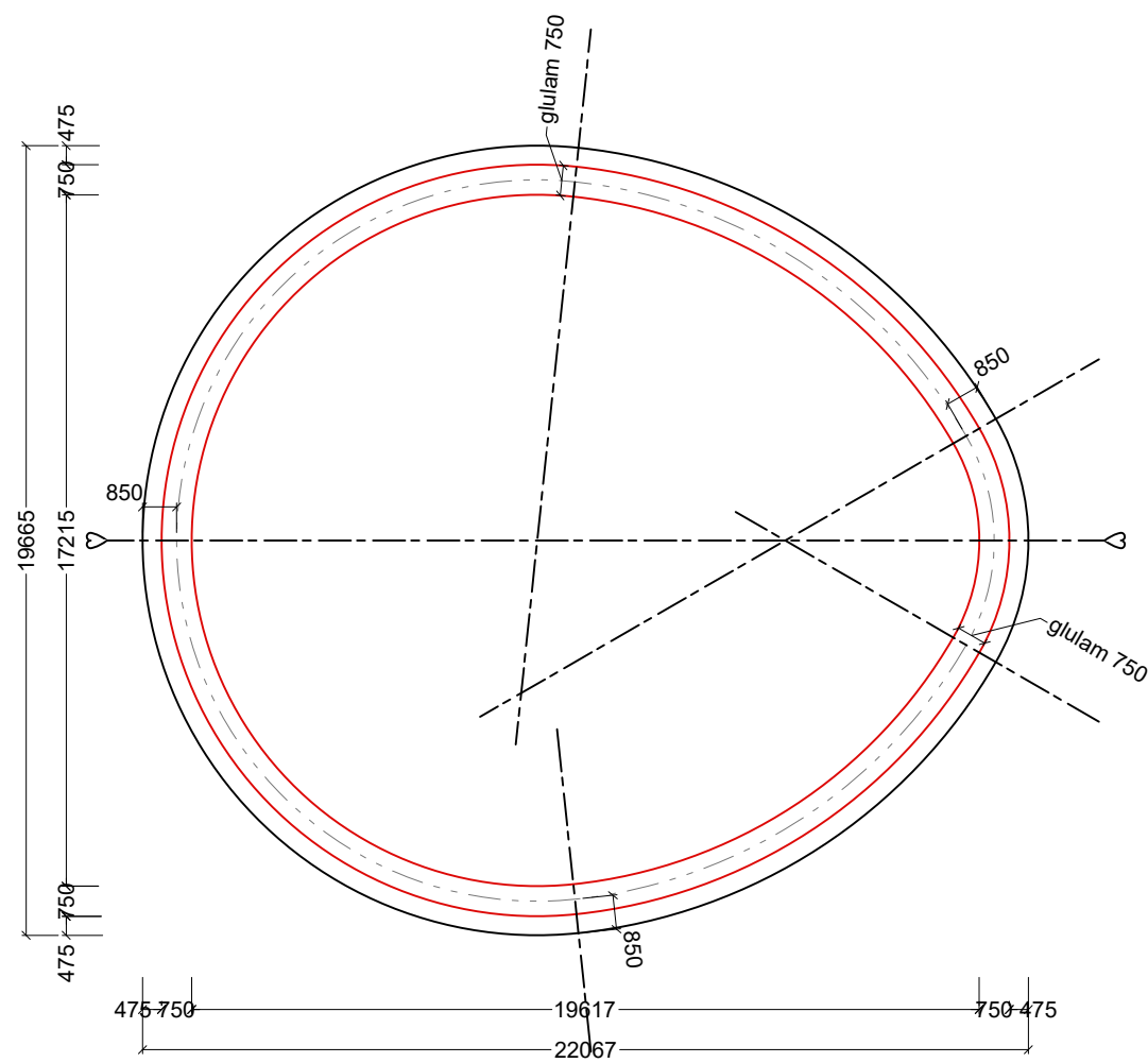
Burðarsúlur sem bera þakið á Bauginum. Stærðir límtréssúlna breidd:750 x hæð:600mm
