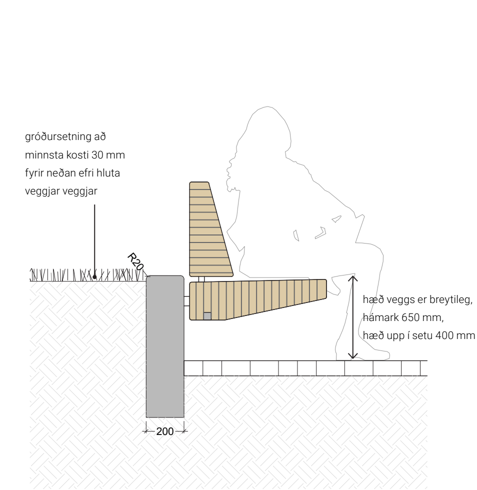
SNID A-A' Veggur 4 á hæsta punkti með bekk staðsettan að ofan
