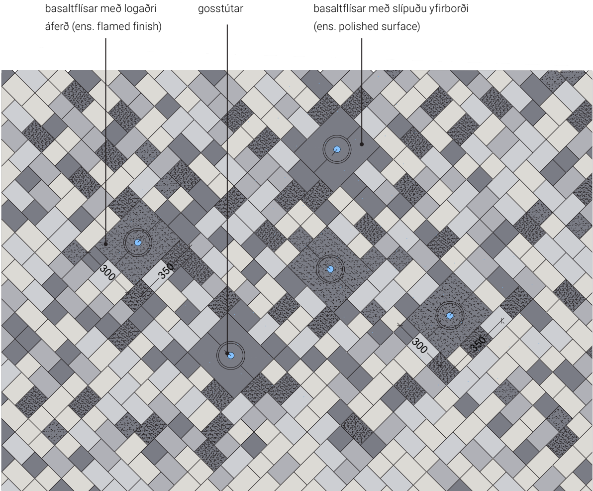
Gosstútar - basaltflísar settar inn gangstéttarhellna mælikvarði 1:200
