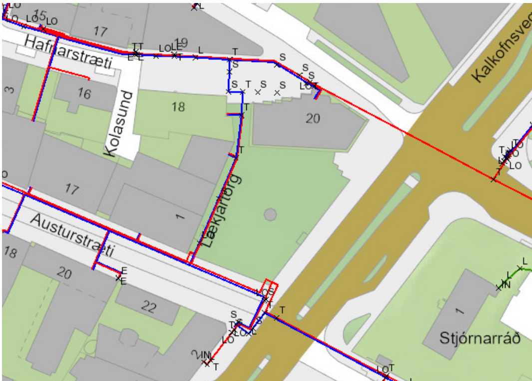
HEITAVATNSLAGNIR
