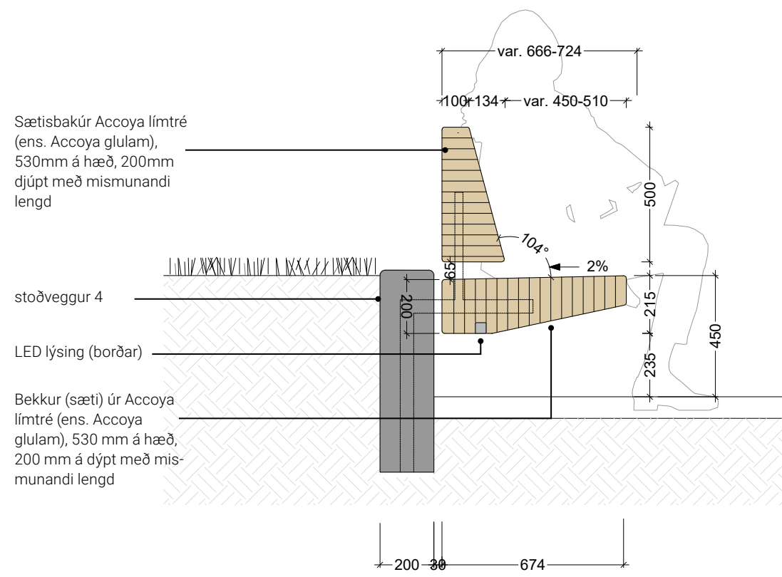
ÁSÝND FRÁ HLIÐ 1
