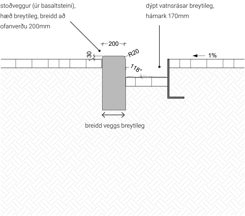
SECTION A-A' Veggur þar sem farið er yfir vatn
