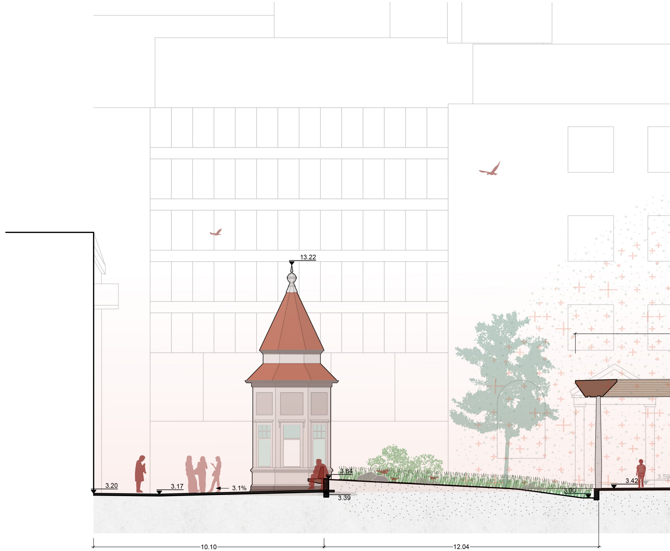
SNID B-B mælikvarði 1:100
