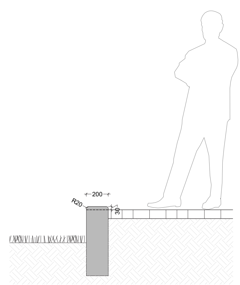
SNID C-C' Veggur 4 þar sem gróðurbeð er innfellt fyrir neðan vegg
