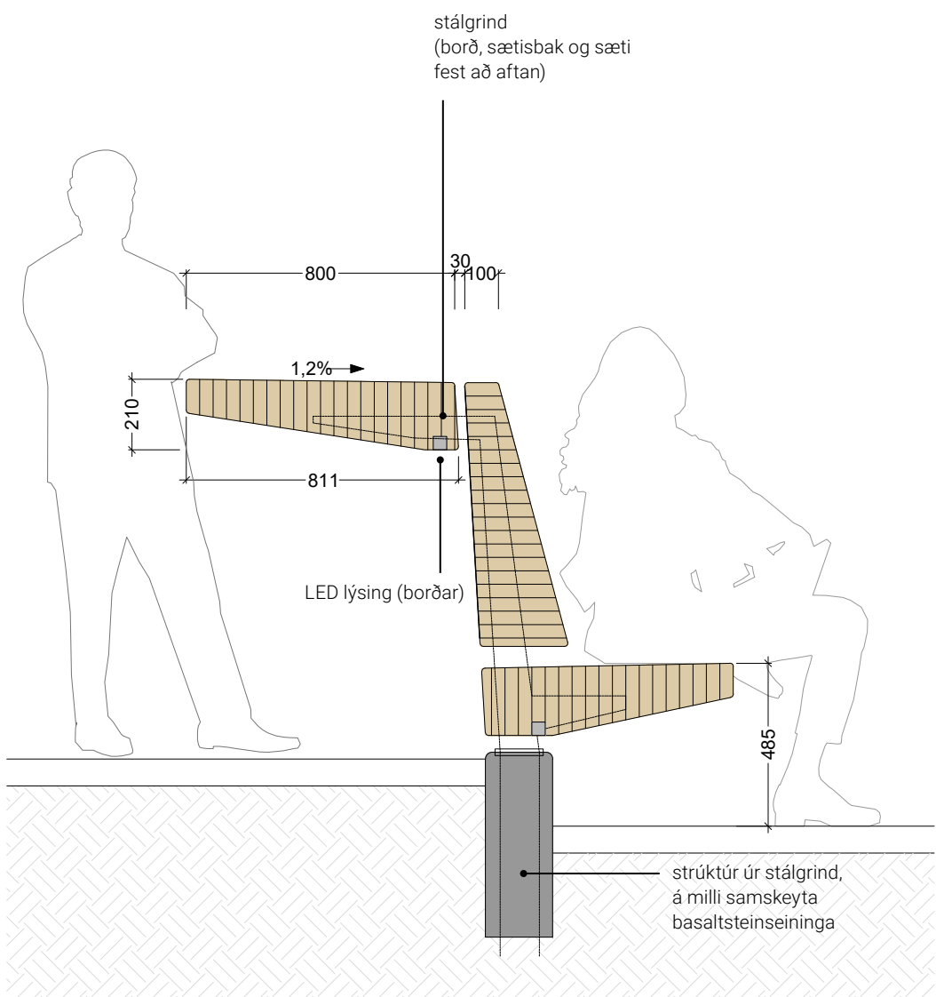
SNÍÐ A-A' Bekkur á breiðasta stað
