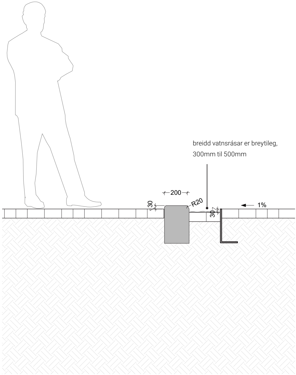
SNID C-C' Veggur við norðurenda
