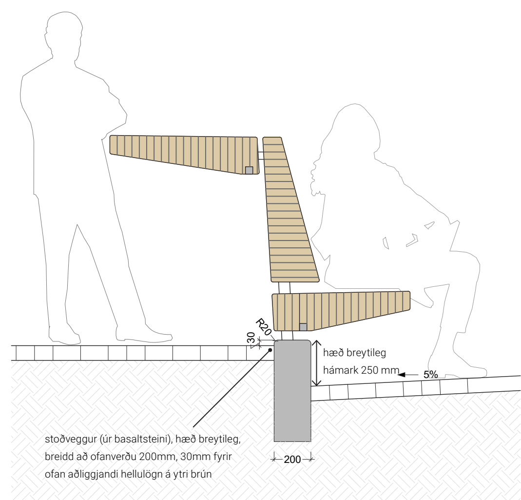
SNID A-A' Veggur 3 á hæsta punkti með bekk staðsettan að ofan
