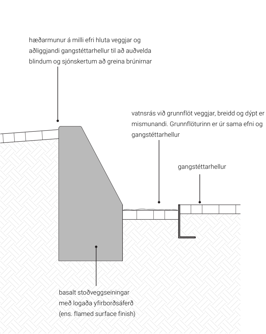
VEGGUR 1 Hallandi veggur með vatnsrás í grunnfleti
