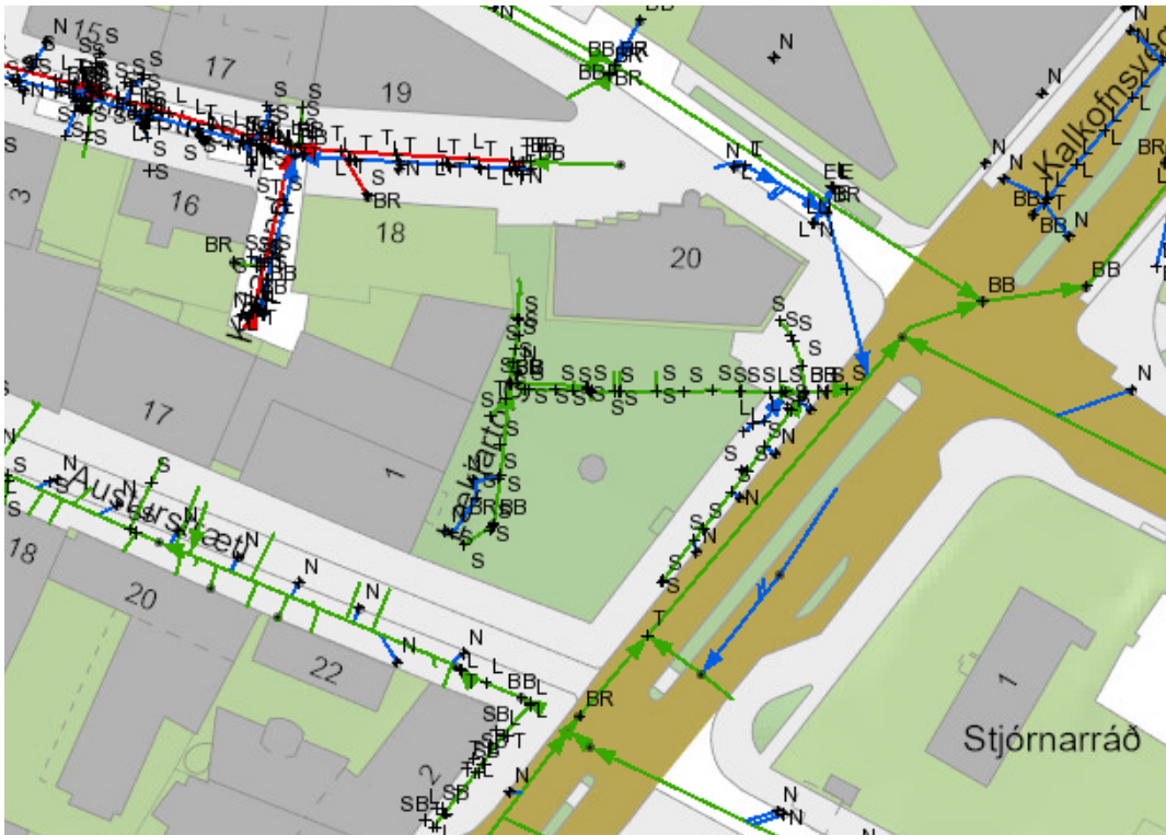
FRÁVEITULAGNIR
