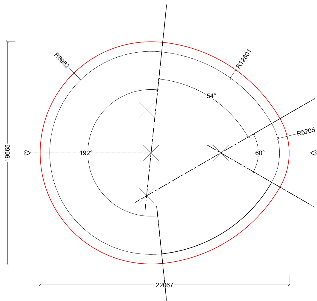
Baugurinn er í formi sporbaugs. Gerður úr 3 mismunandi bogaformum (ens. tangential arcs)
