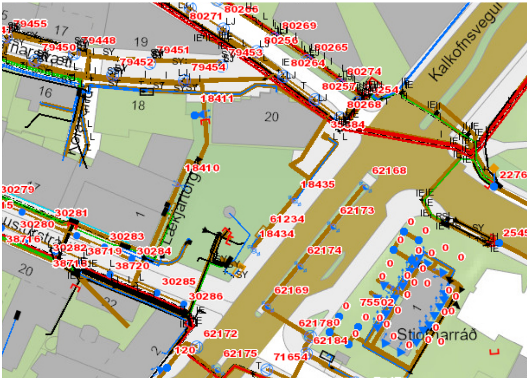
RAFMAGNSLAGNIR
