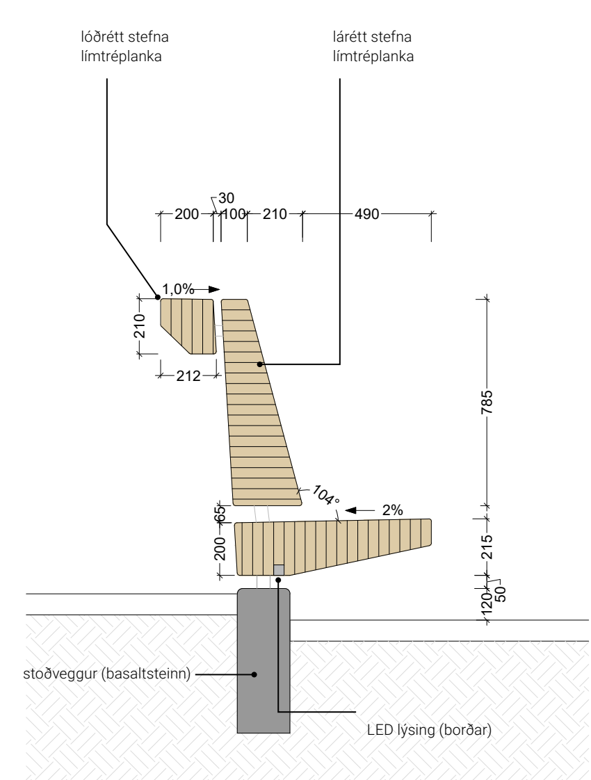
ÁSÝND FRÁ HLÍÐ Bekkur á þrengsta stað
