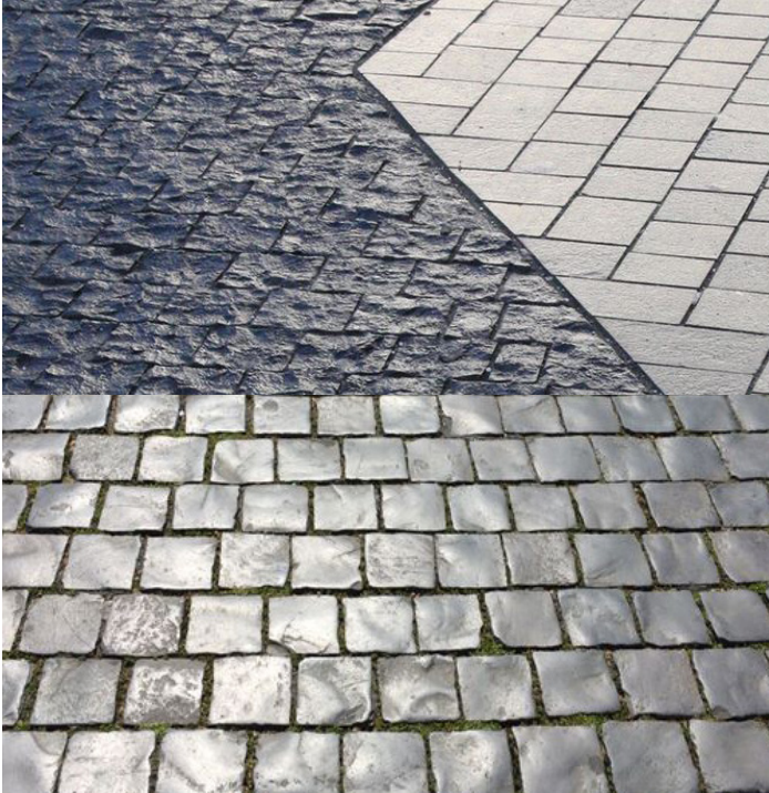
Basaltsteinar með brotnu (efst til vinstri), brenndu/loguðu (efst til hægri) og slípuðu (neðst) yfirborði
