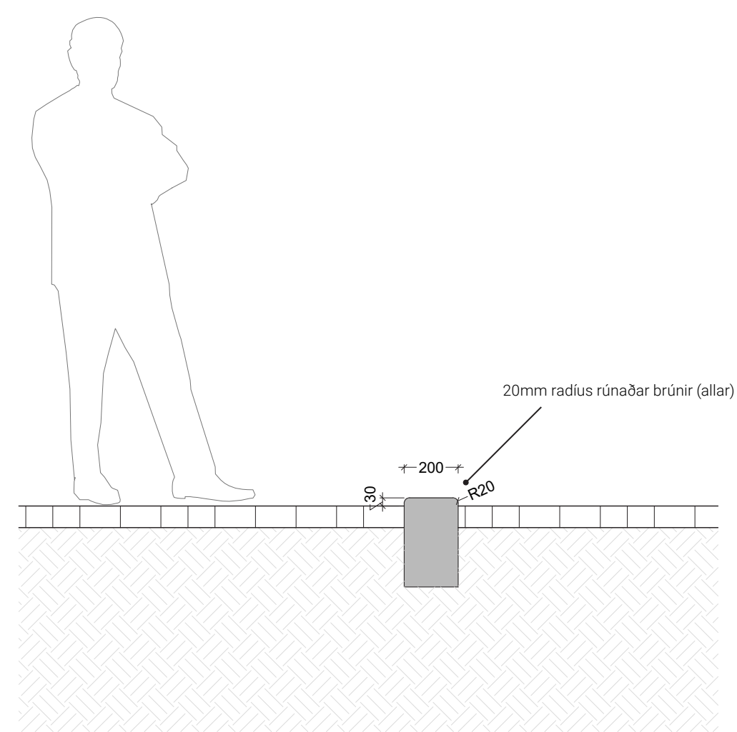
SNID B-B' Veggur 3 á lægstu punktum á hvorum enda
