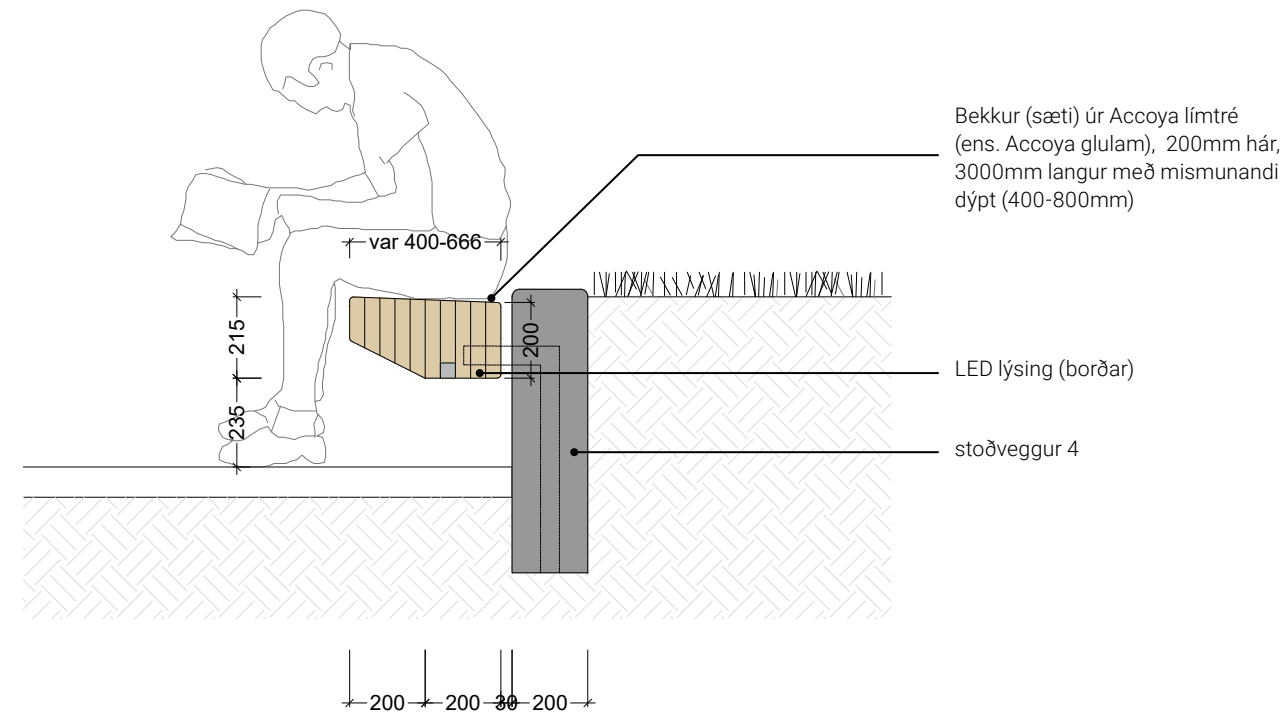
ÁSÝND FRÁ HLIÐ 2
