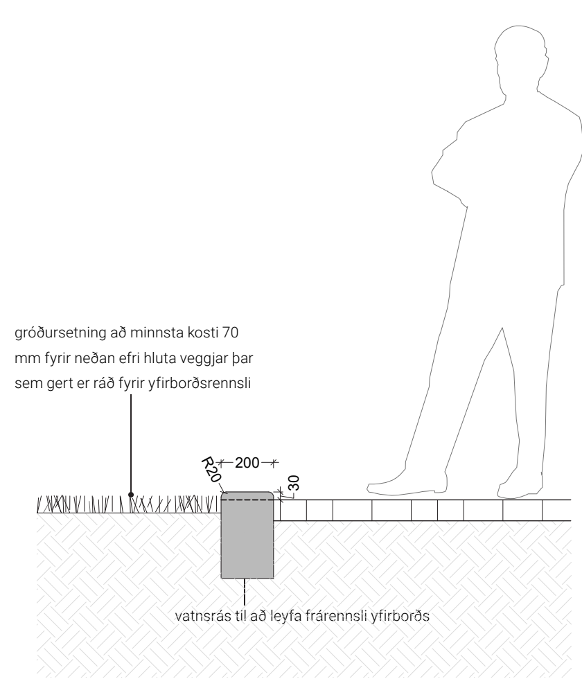
SNID B-B' Veggur 4 á lágsta punkti
