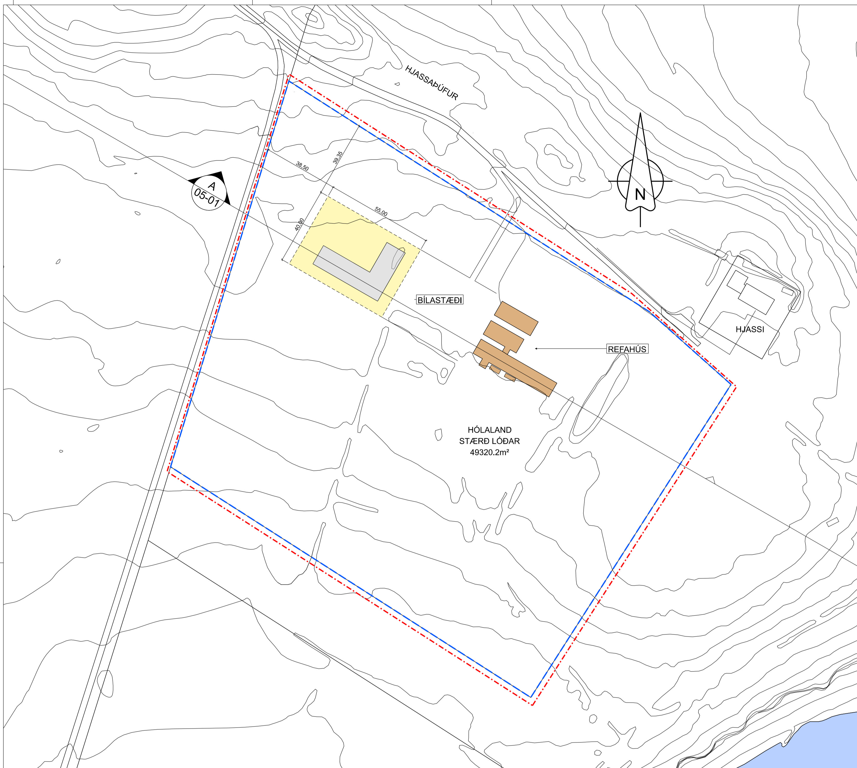
1 DEILISKIPULAG 1:1000
