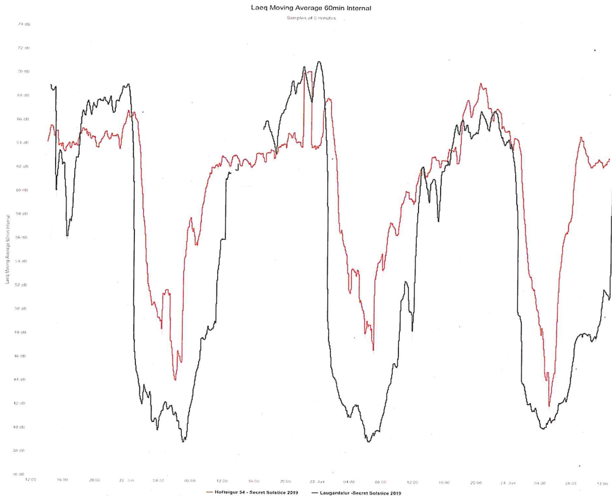
Mynd 1 Myndin sýnir hljóðstig á báðum hljóðmælum á meðan hátíðin stóð yfir 21-23. júní
