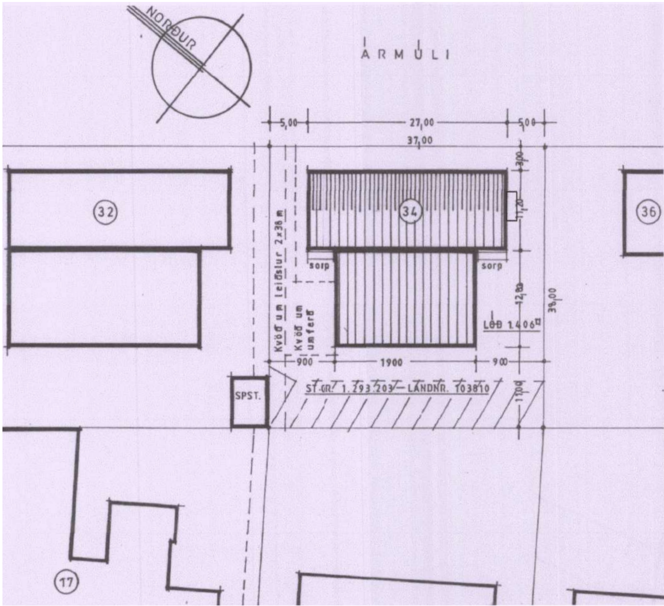
Afstöðumynd 1:500
