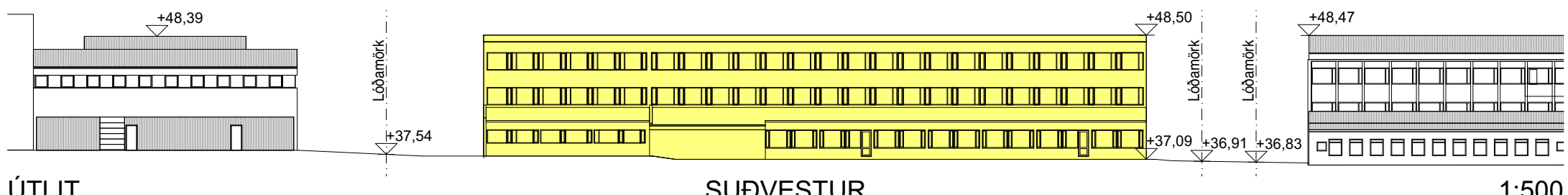
ÚTLIT SUDVESTUR
